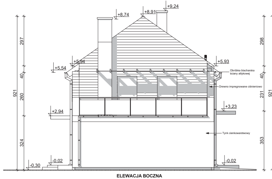
ELEWACJA BOCZNA
