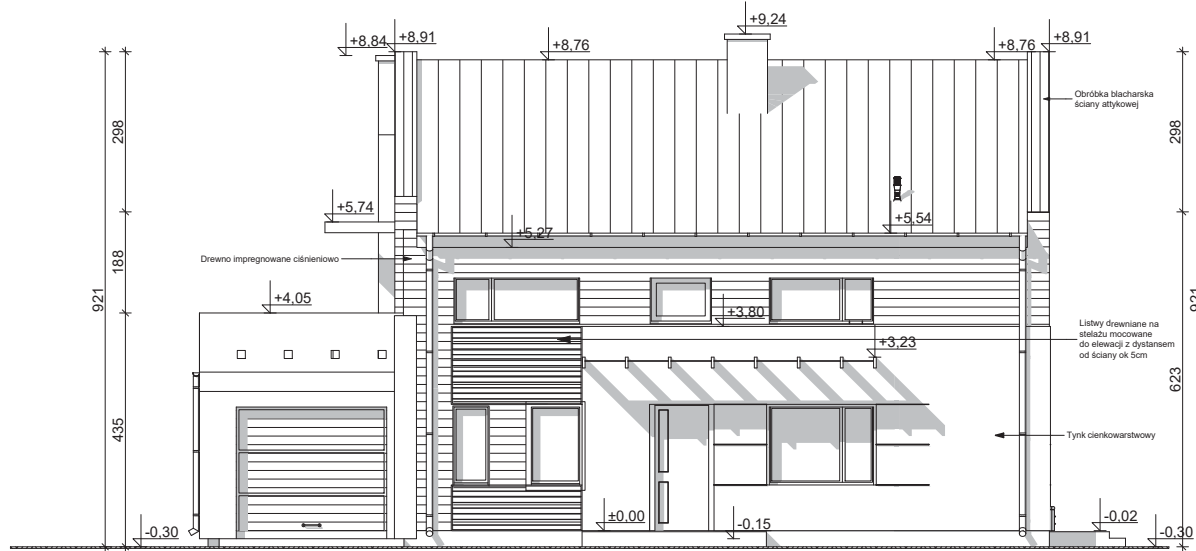
ELEWACJA FRONTOWA
