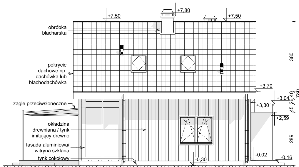
ELEWACJA BOCZNA
