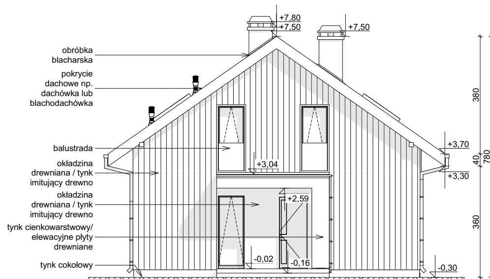
ELEWACJA FRONTOWA
