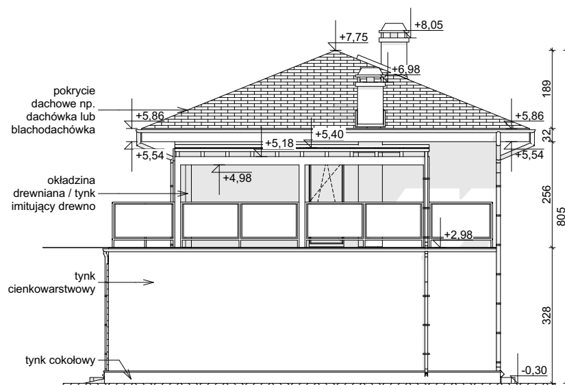
ELEWACJA BOCZNA
