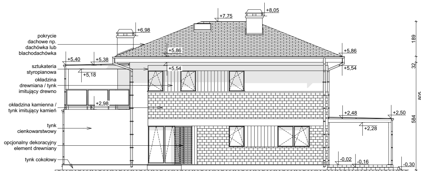
ELEWACJA OGRODOWA
