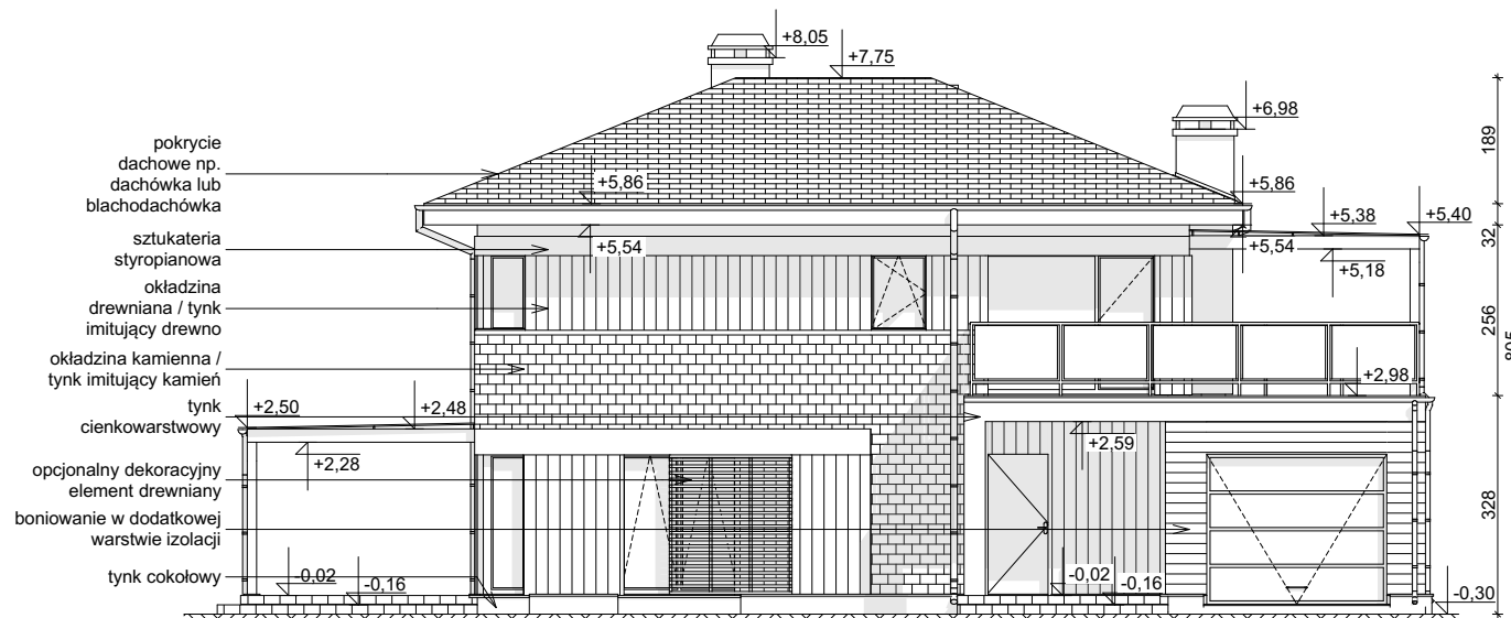
ELEWACJA FRONTOWA
