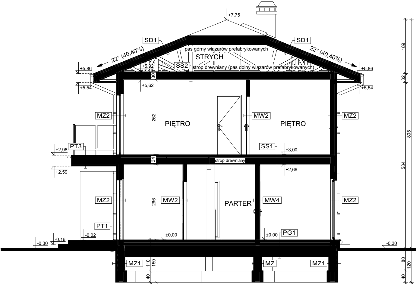
PRZEKRÓJ B-B
