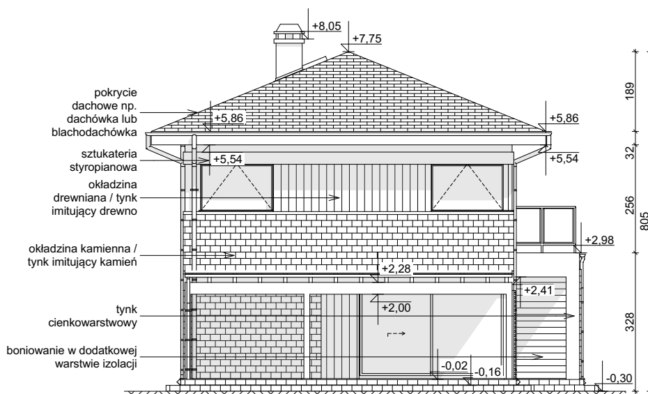
ELEWACJA BOCZNA
