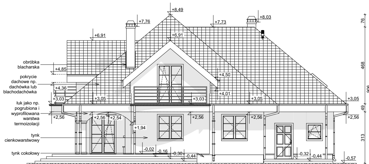
ELEWACJA OGRODOWA
