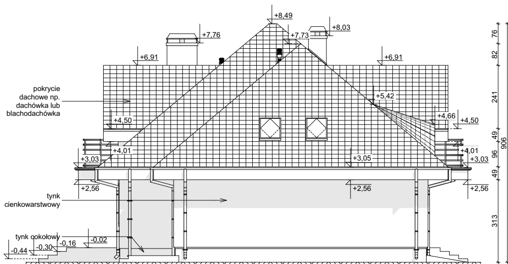
ELEWACJA BOCZNA
