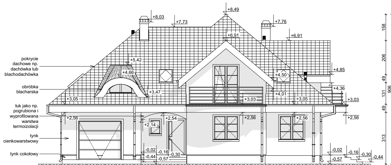
ELEWACJA FRONTOWA
