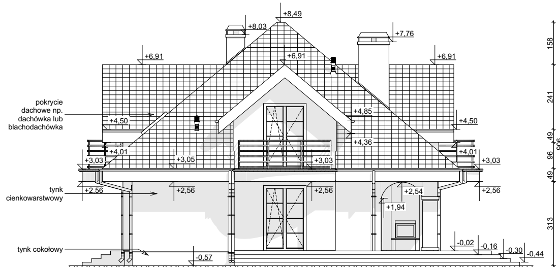
ELEWACJA BOCZNA
