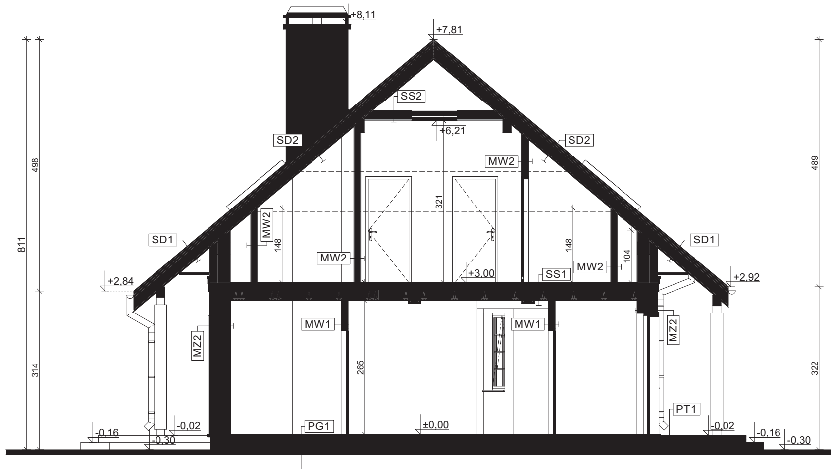
PRZEKRÓJ B-B
