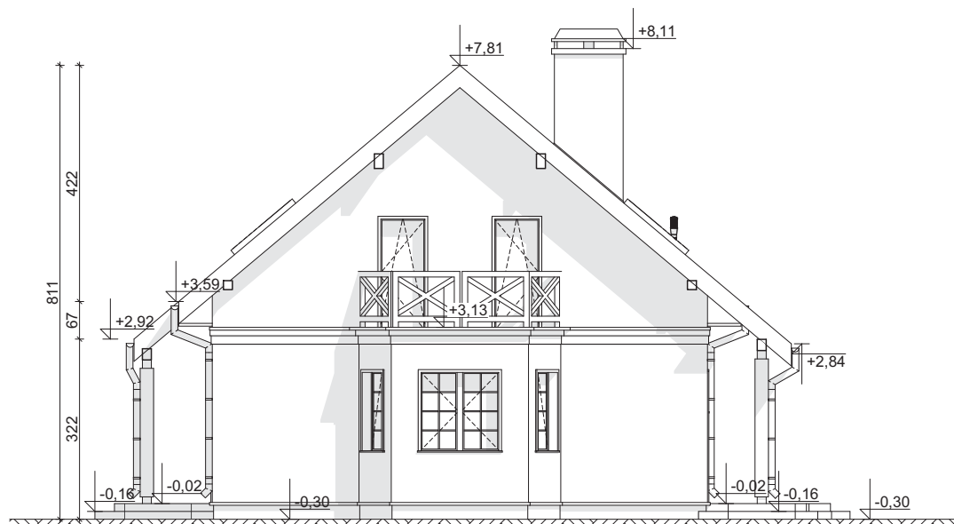
ELEWACJA BOCZNA
