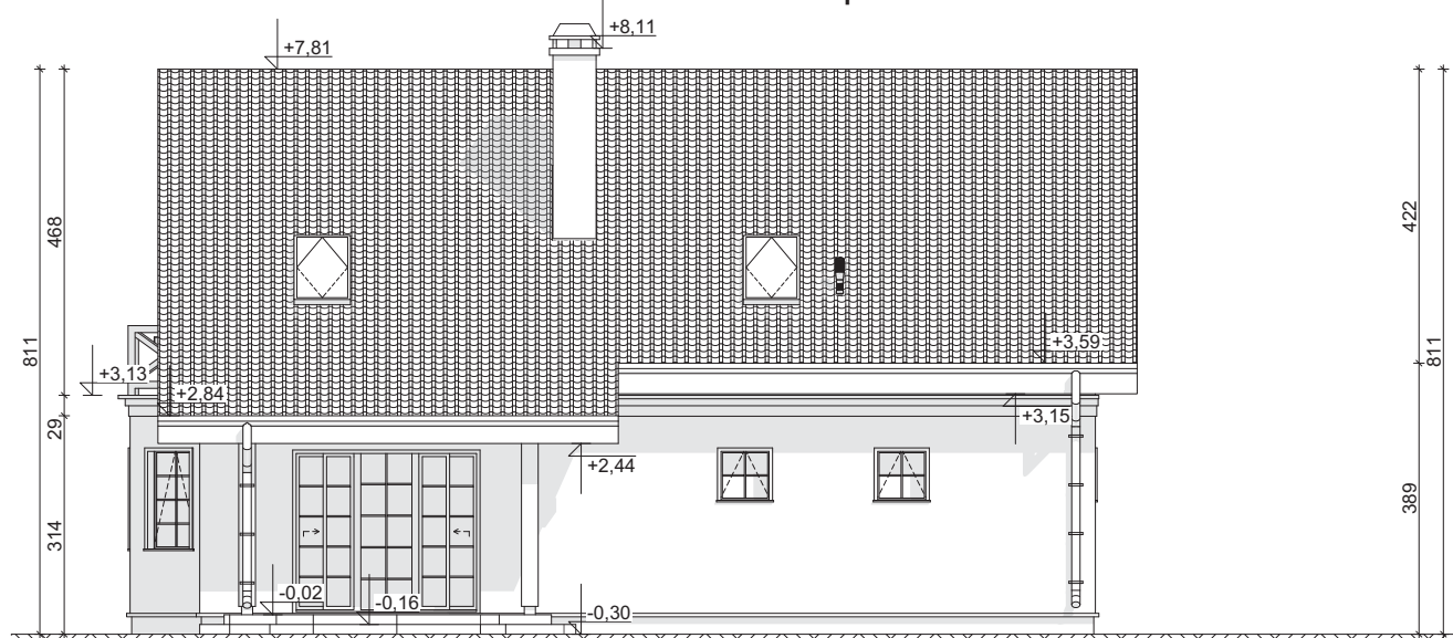
ELEWACJA OGRODOWA
