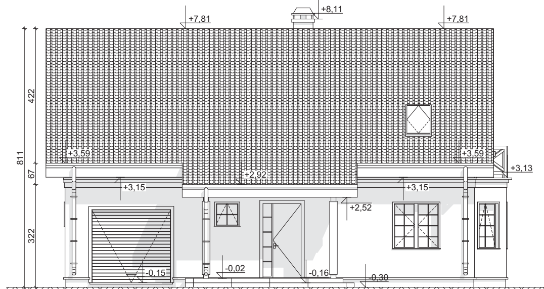
ELEWACJA FRONTOWA
