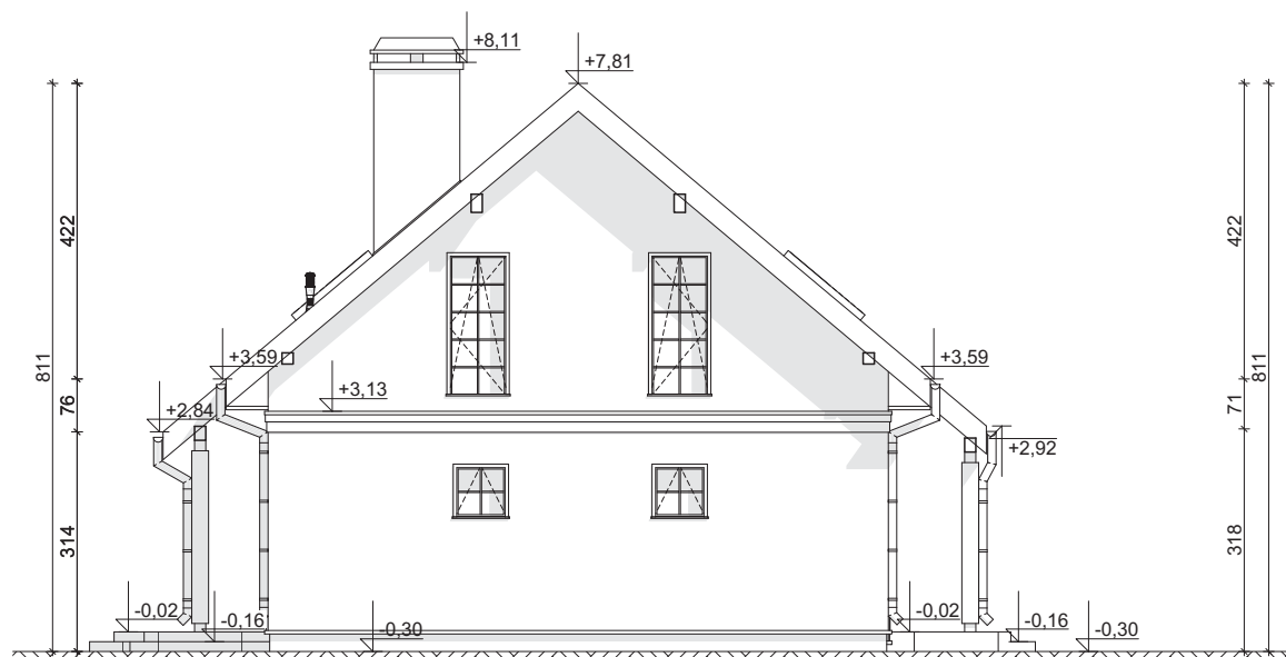
ELEWACJA BOCZNA
