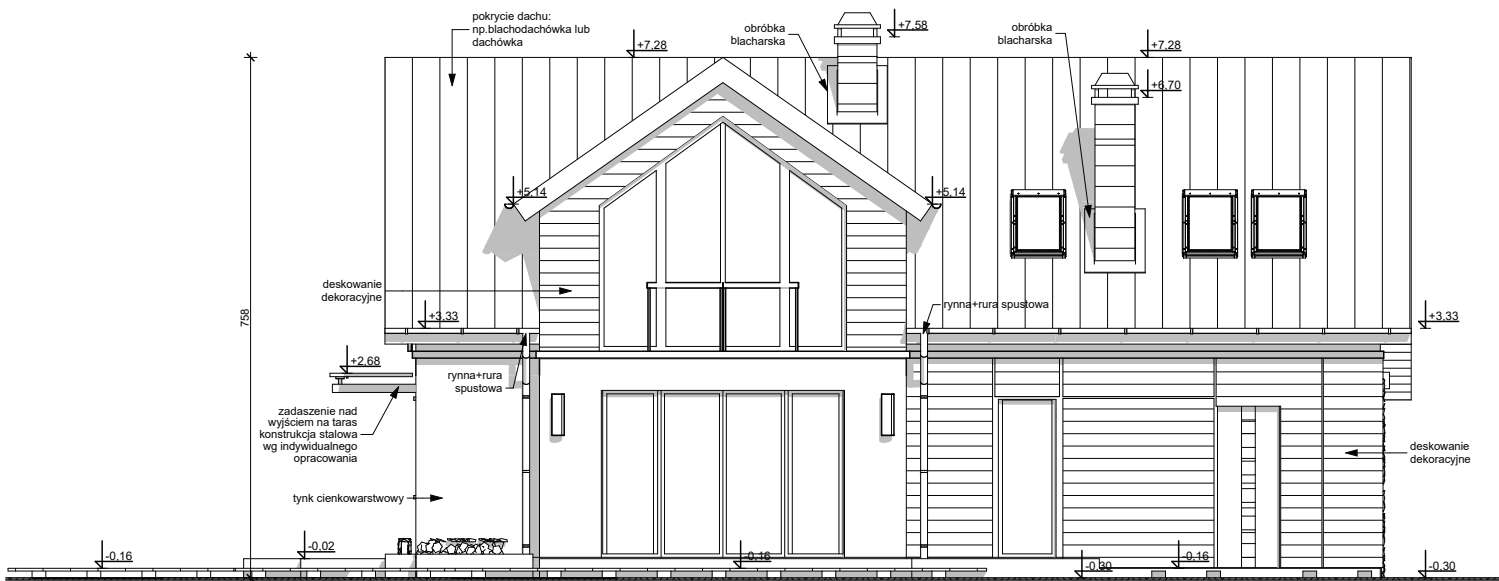
ELEWACJA TYLNA
