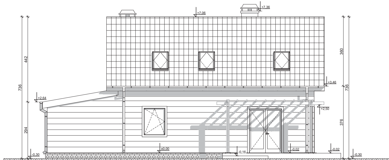
ELEWACJA TYLNA
