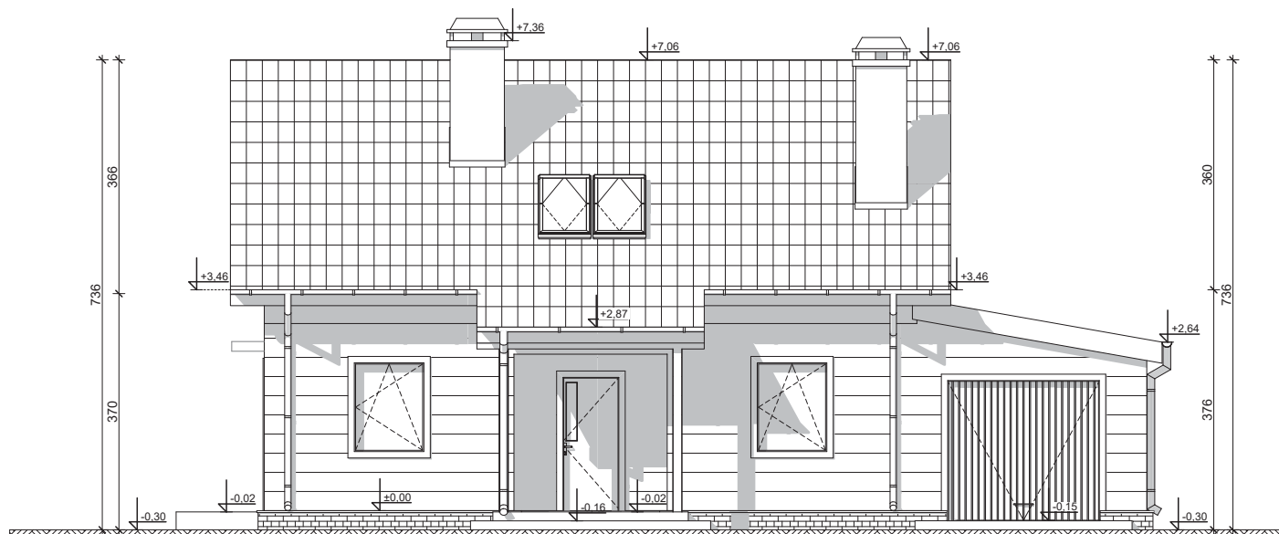
ELEWACJA FRONTOWA
