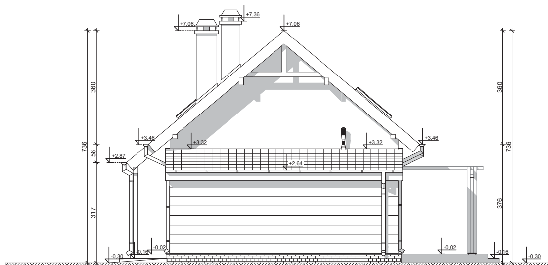
ELEWACJA BOCZNA
