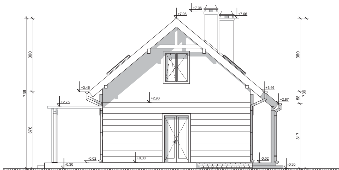
ELEWACJA BOCZNA
