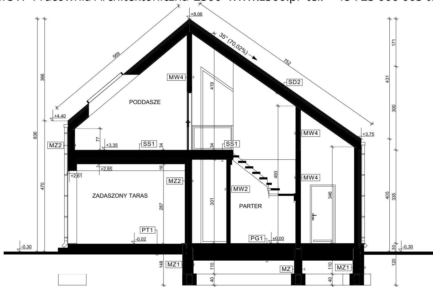
PRZEKRÓJ A-A
