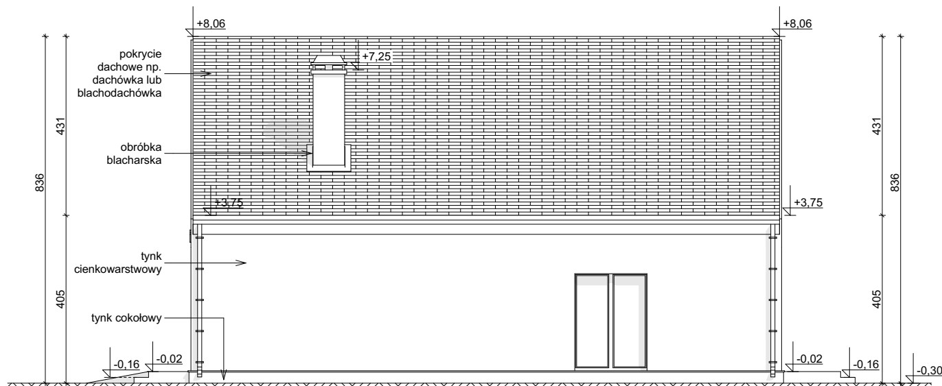
ELEWACJA BOCZNA
