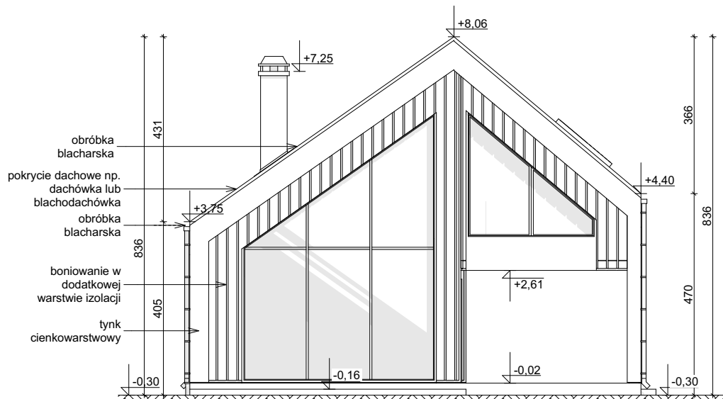
ELEWACJA OGRODOWA
