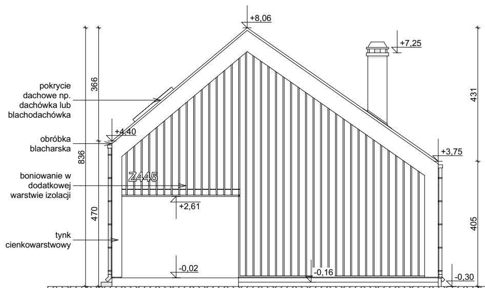
ELEWACJA FRONTOWA
