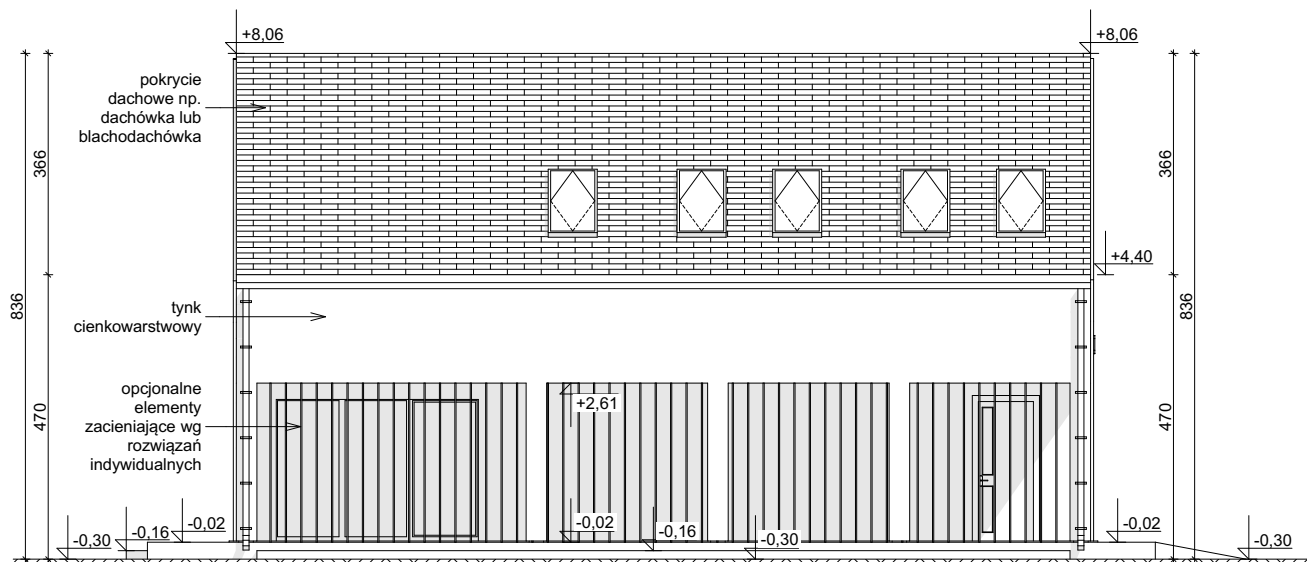
ELEWACJA BOCZNA
