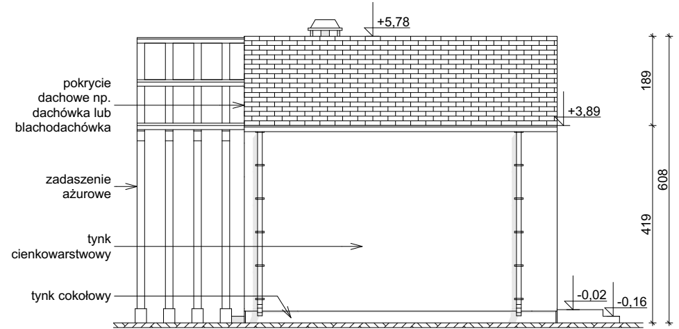
ELEWACJA BOCZNA
