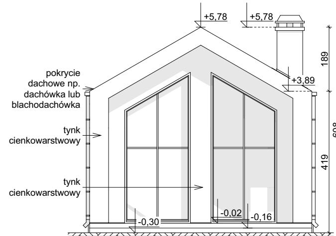
ELEWACJA OGRODOWA
