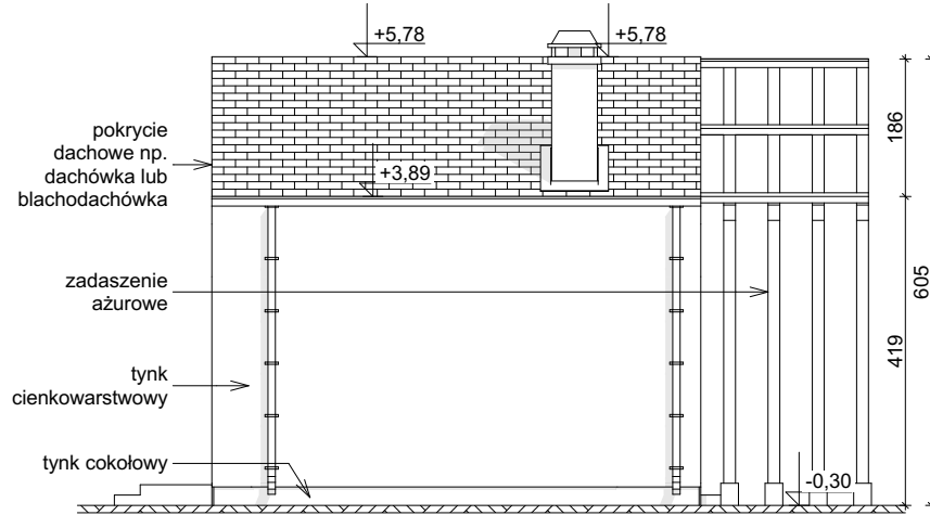
ELEWACJA BOCZNA
