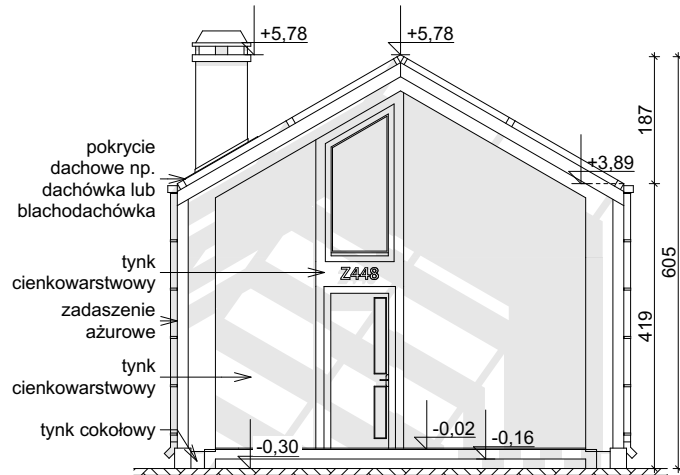
ELEWACJA FRONTOWA
