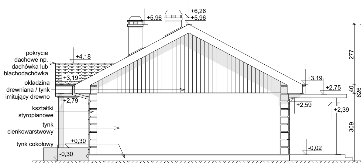
ELEWACJA BOCZNA
