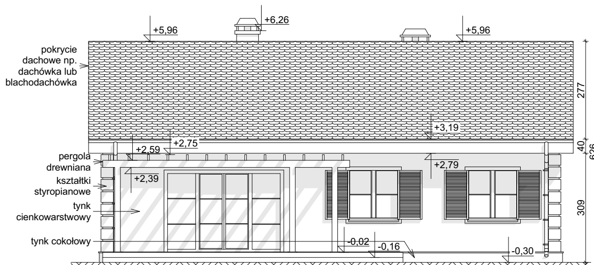
ELEWACJA OGRODOWA
