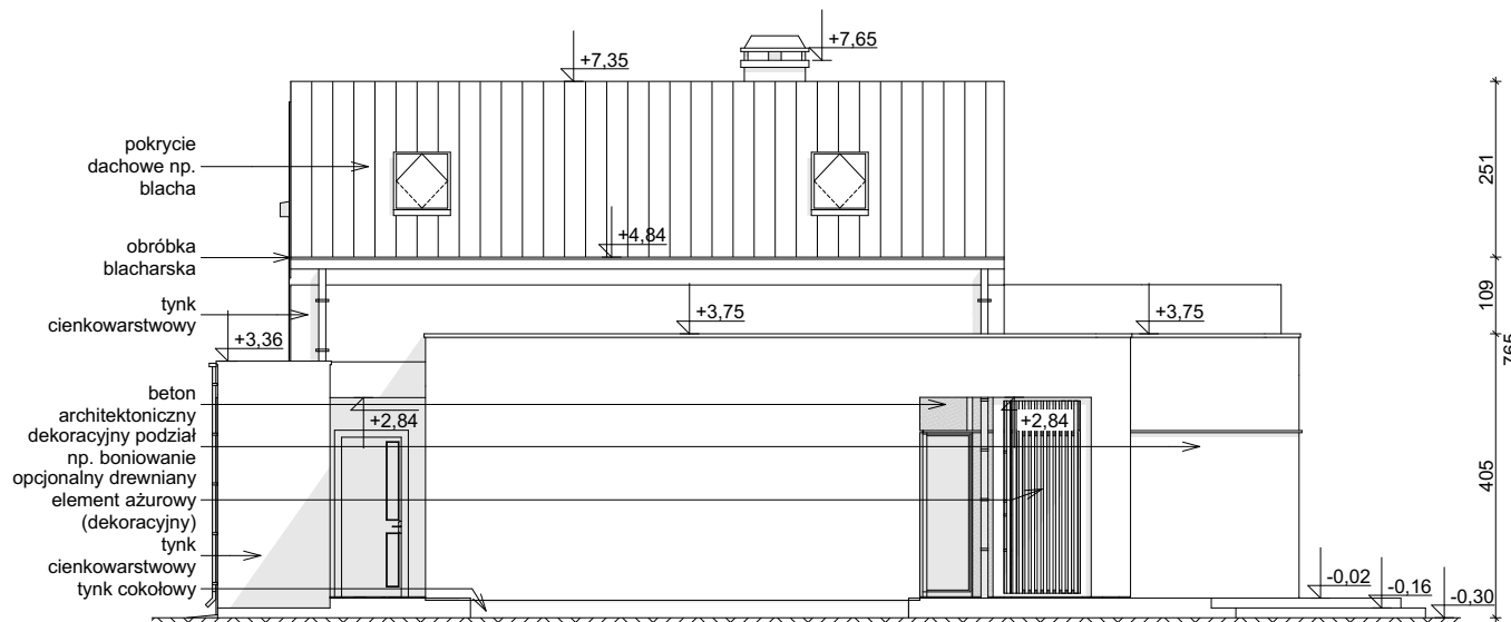
ELEWACJA BOCZNA
