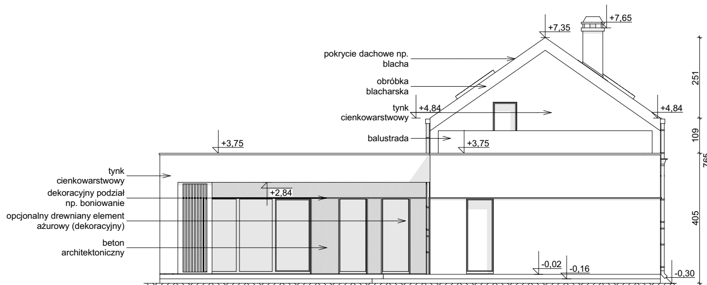
ELEWACJA OGRODOWA
