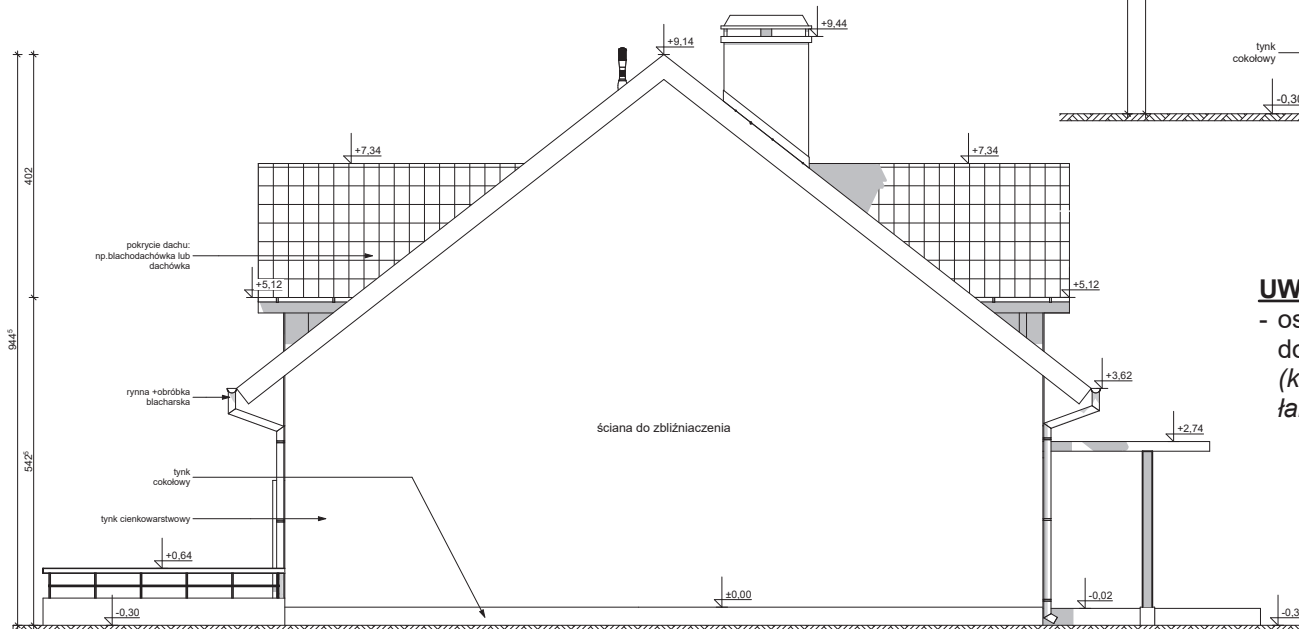
ELEWACJA BOCZNA
