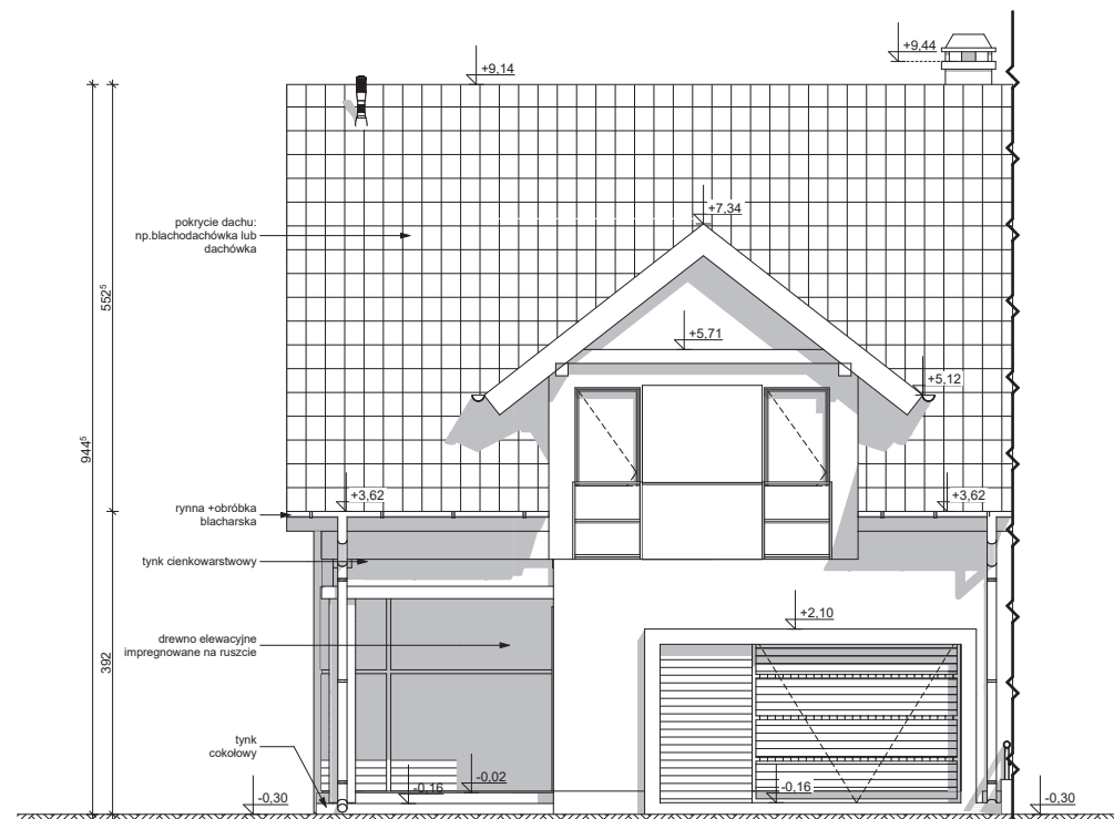
ELEWACJA FRONTOWA
