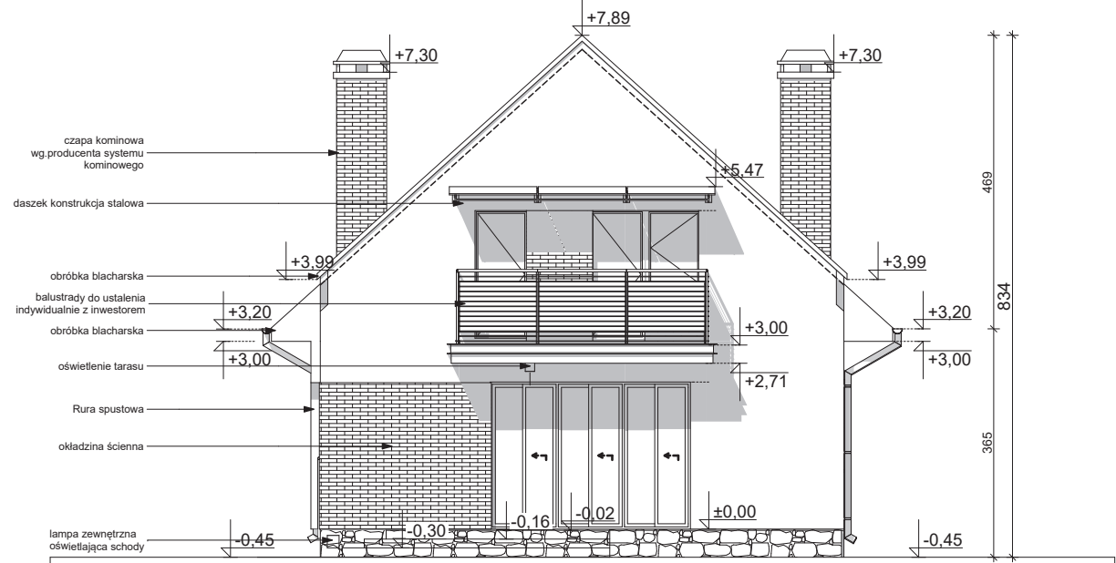
ELEWACJA TYLNA
