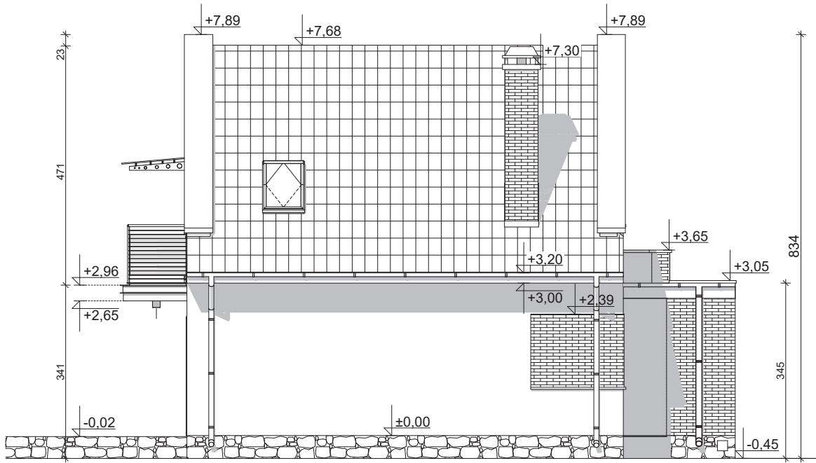
ELEWACJA BOCZNA
