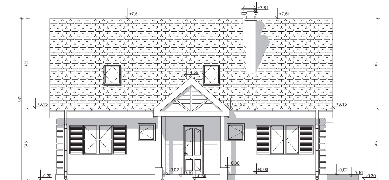
ELEWACJA FRONTOWA
