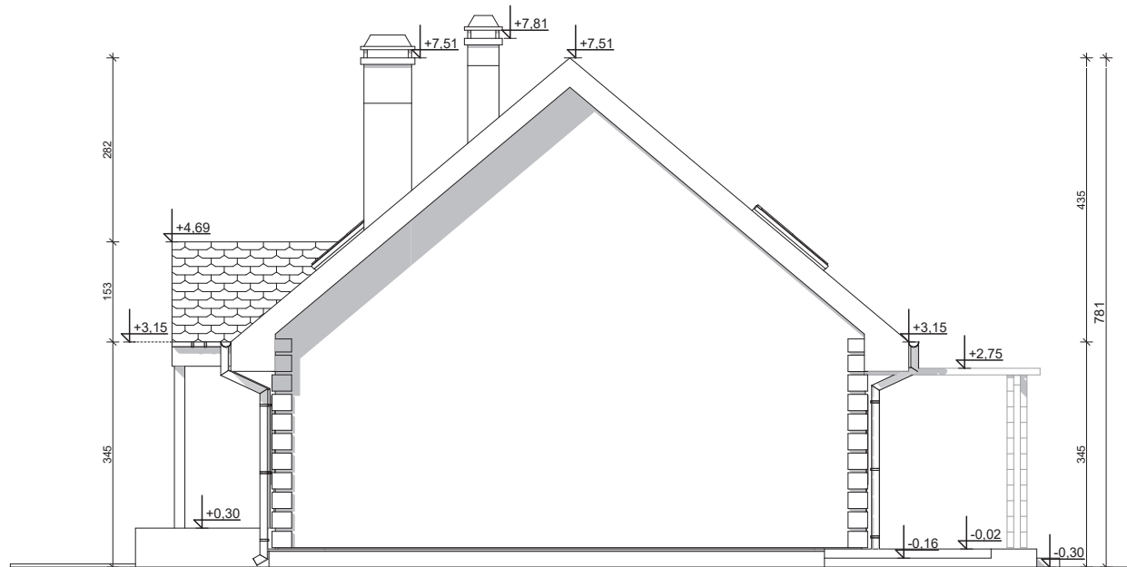
ELEWACJA BOCZNA
