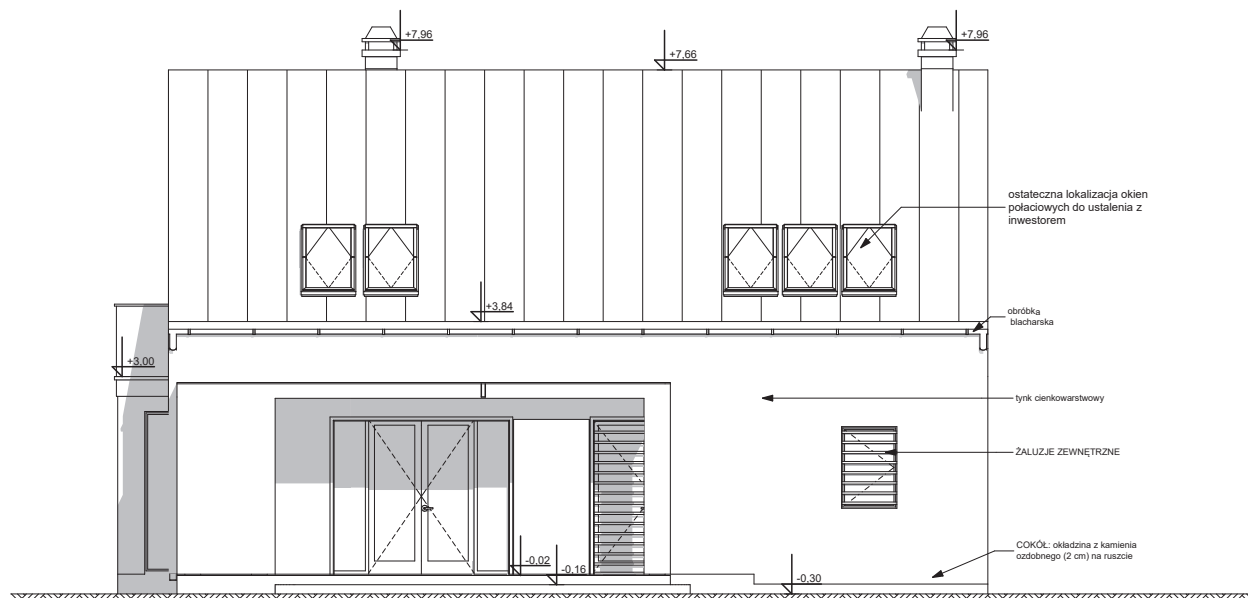
Elewacja tylna
