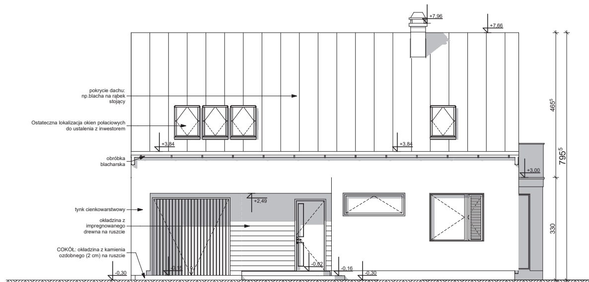
Elewacja frontowa
