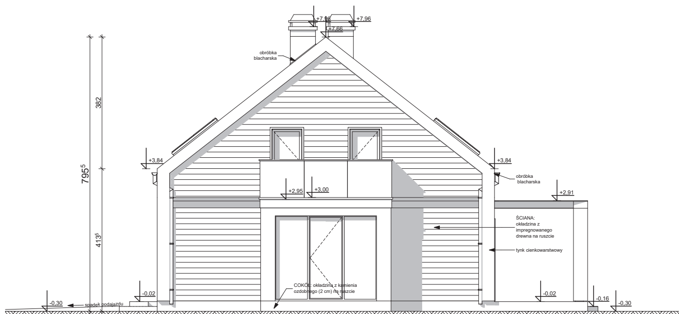
Elewacja boczna
