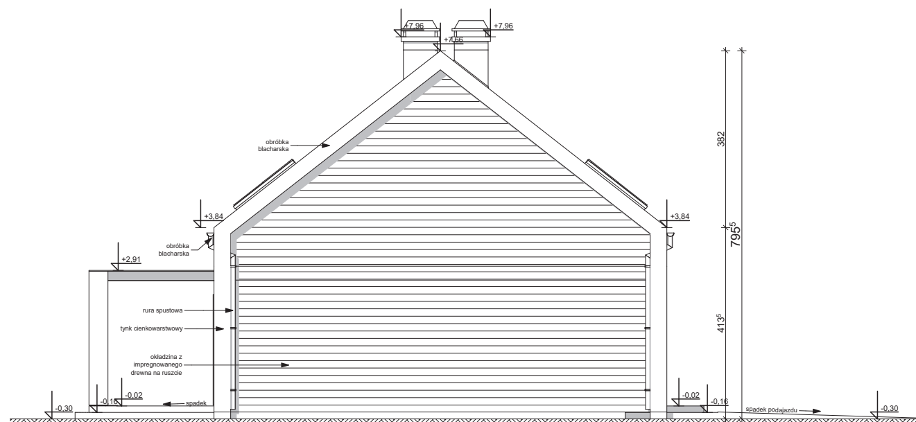
Elewacja boczna
