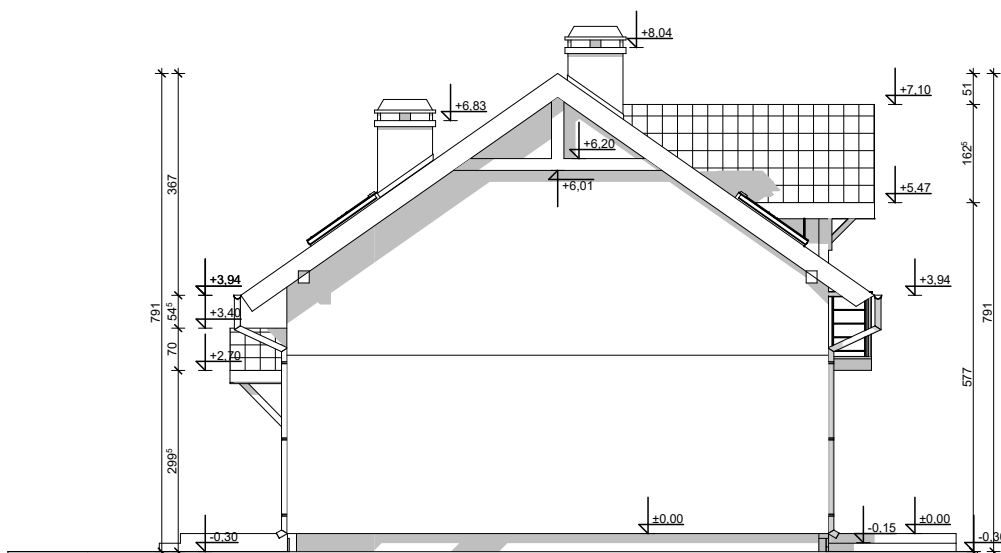
Elewacja boczna
