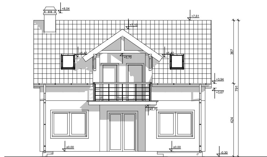
Elewacja tylna
