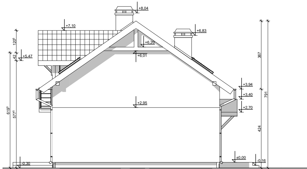
Elewacja boczna
