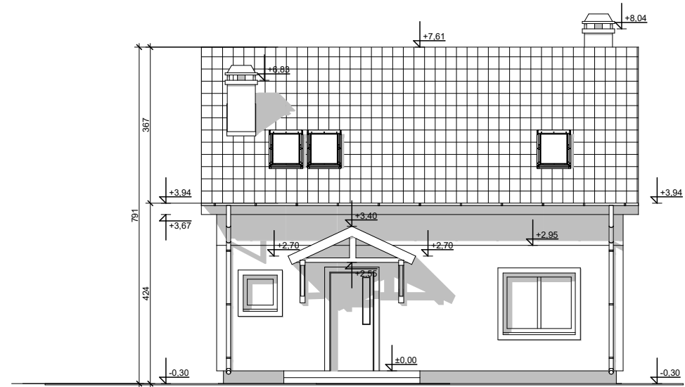
Elewacja frontowa
