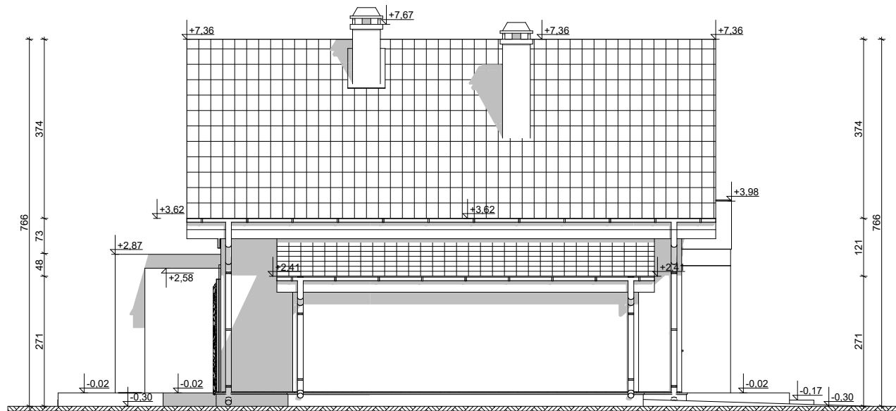
ELEWACJA BOCZNA
