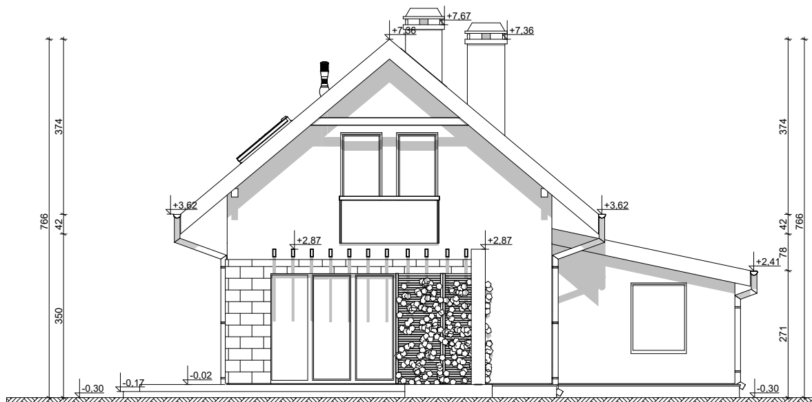
ELEWACJA OGRODOWA
