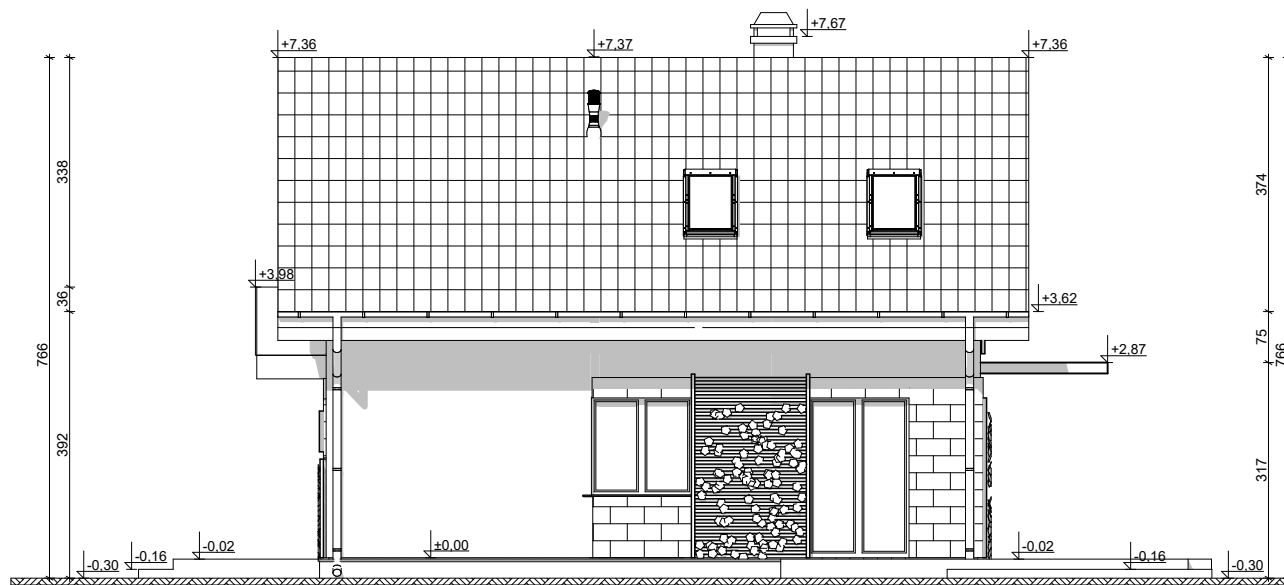
ELEWACJA BOCZNA
