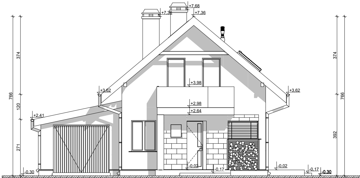
ELEWACJA FRONTOWA
