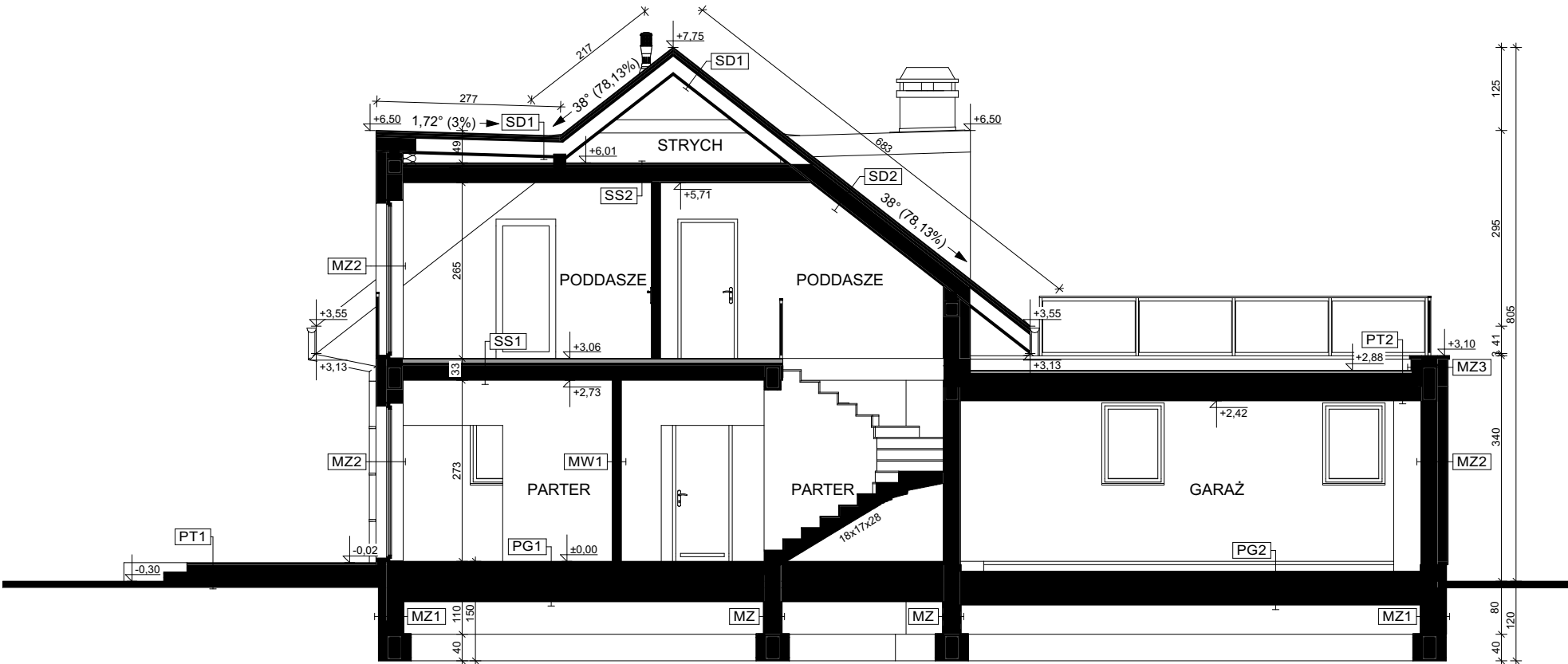
PRZEKRÓJ B-B
