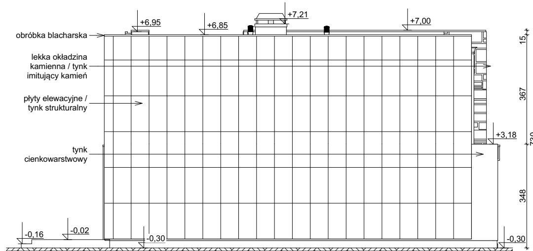
ELEWACJA BOCZNA
