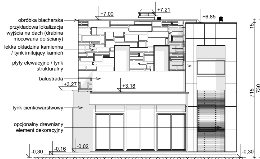
ELEWACJA OGRODOWA
