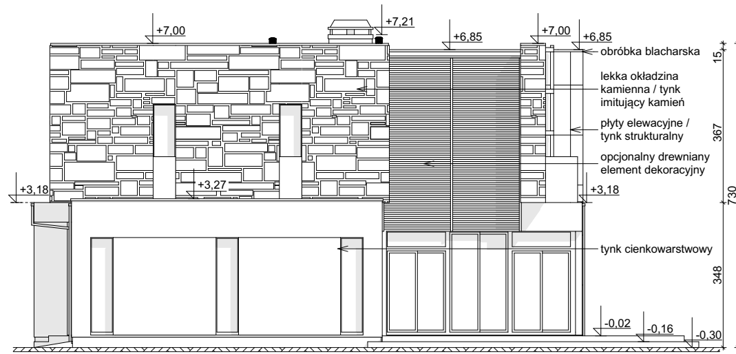
ELEWACJA BOCZNA
