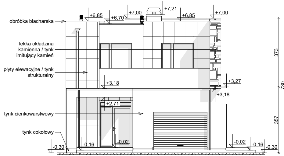
ELEWACJA FRONTOWA
