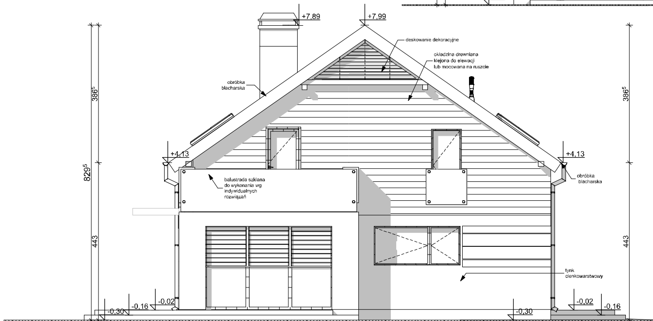
ELEWACJA BOCZNA
