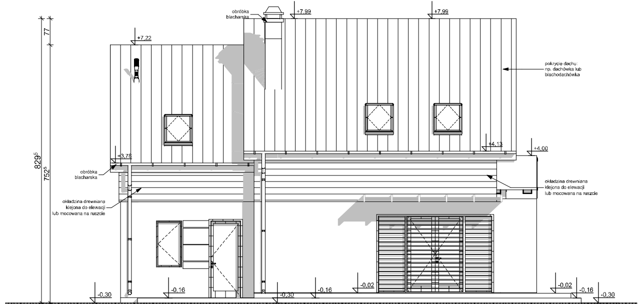
ELEWACJA TYLNA
