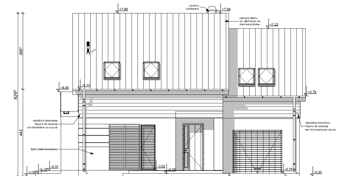
ELEWACJA FRONTOWA
