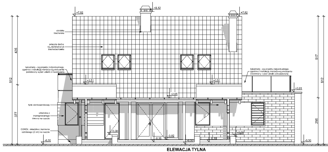
ELEWACJA TYLNA
