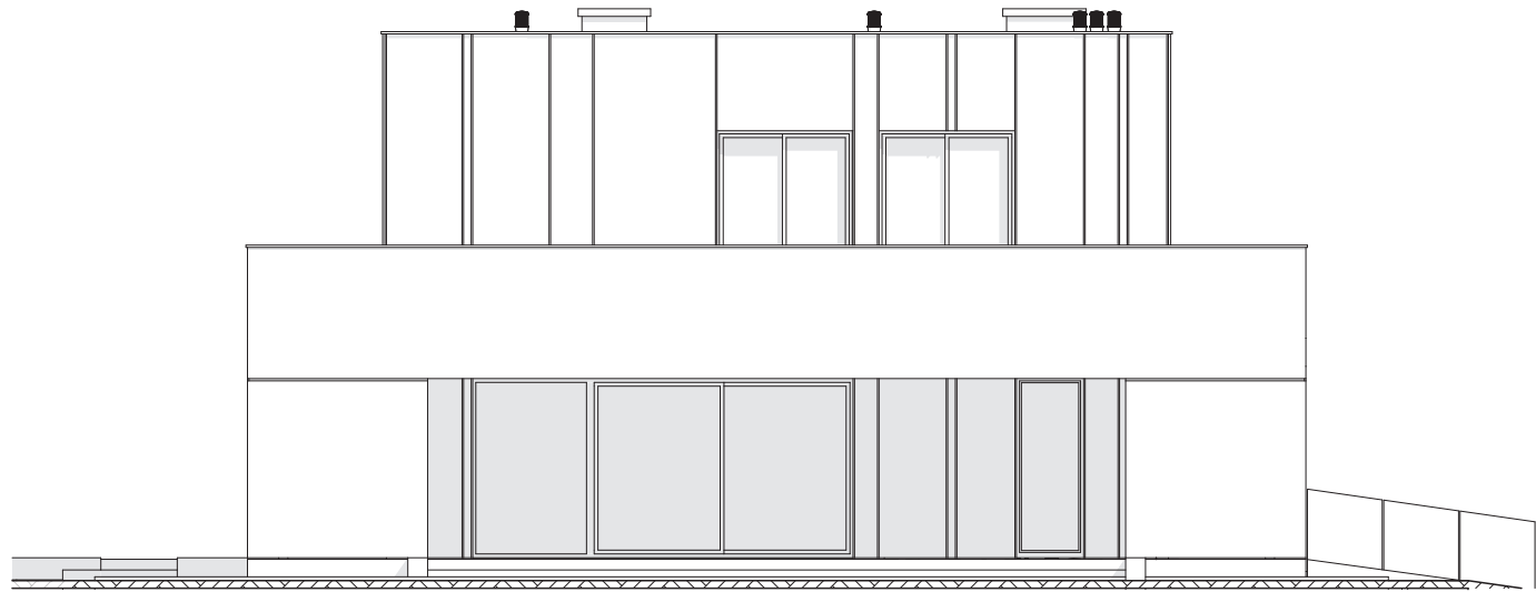
ELEWACJA BOCZNA
