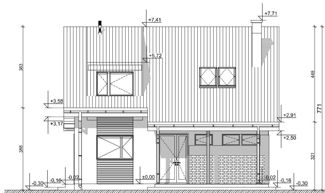
ELEWACJA FRONTOWA
