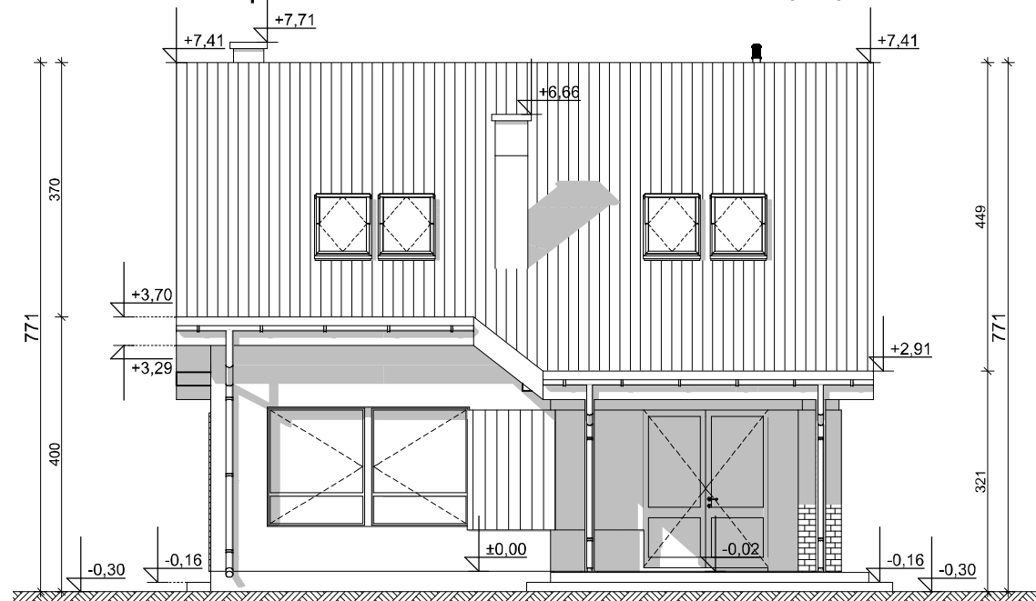
ELEWACJA TYLNA
