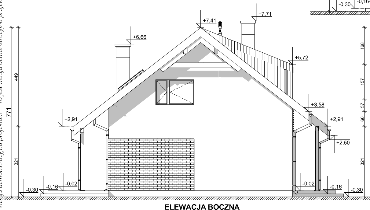
ELEWACJA BOCZNA
