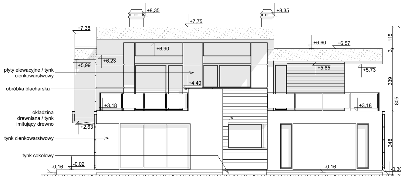
ELEWACJA OGRODOWA
