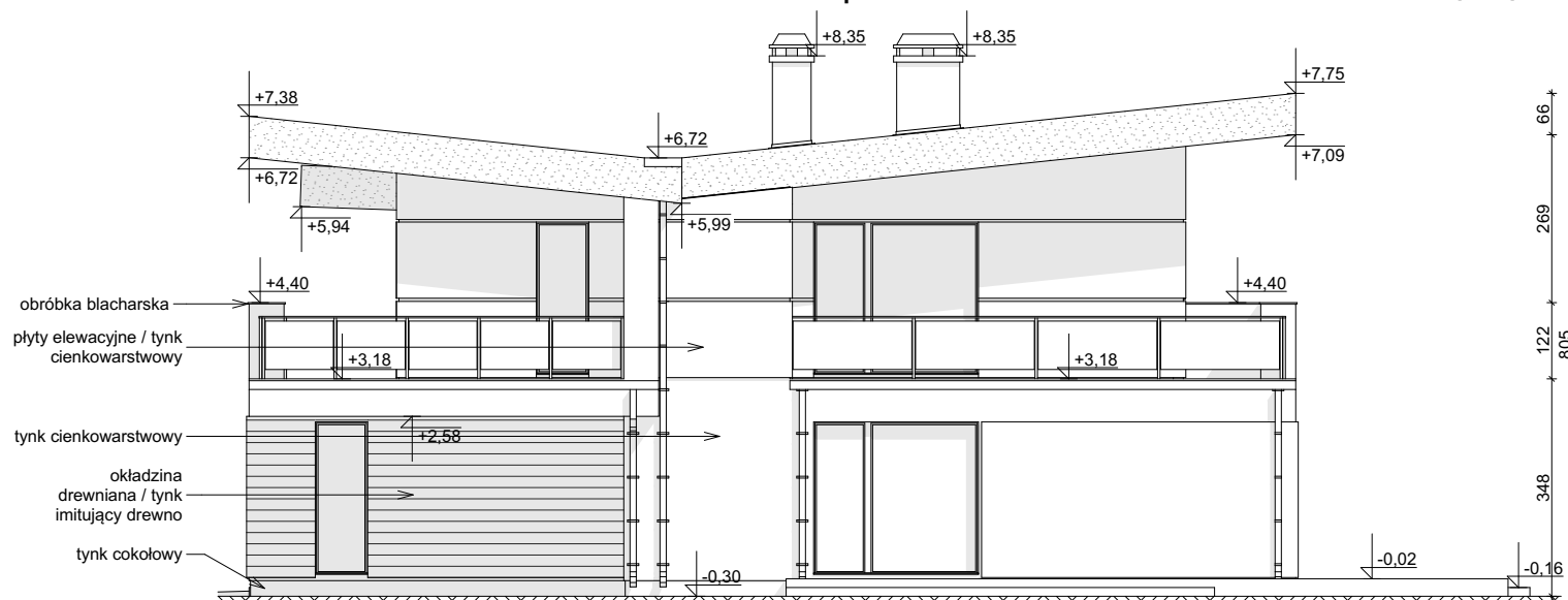
ELEWACJA BOCZNA
