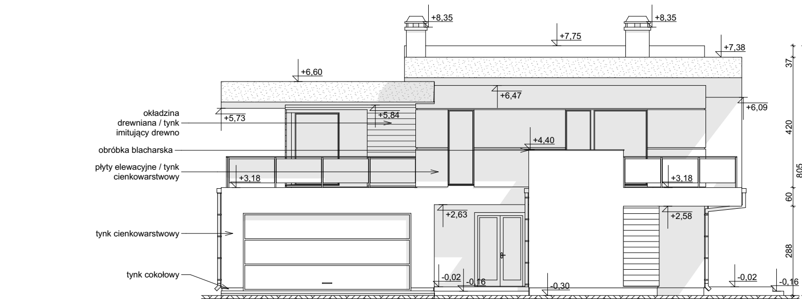
ELEWACJA FRONTOWA
