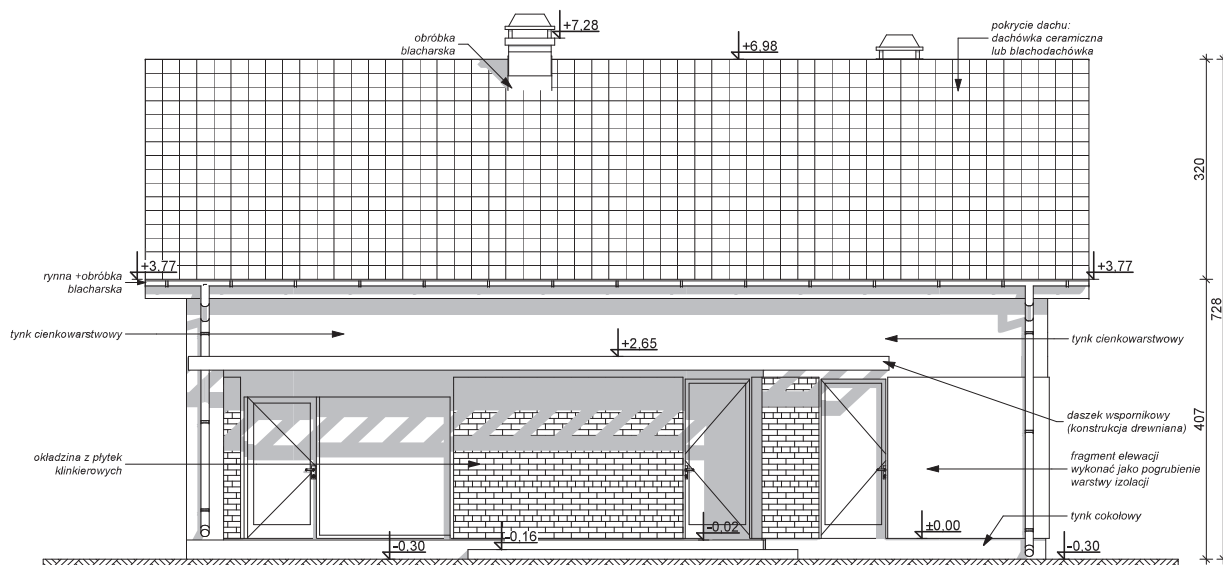
ELEWACJA TYLNA
