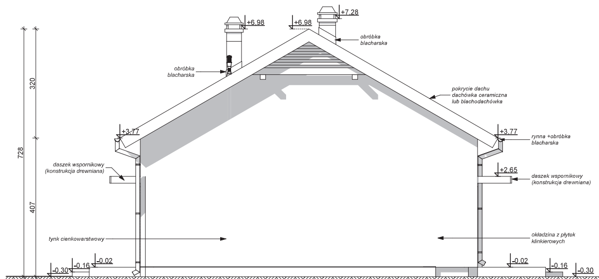
ELEWACJA BOCZNA
