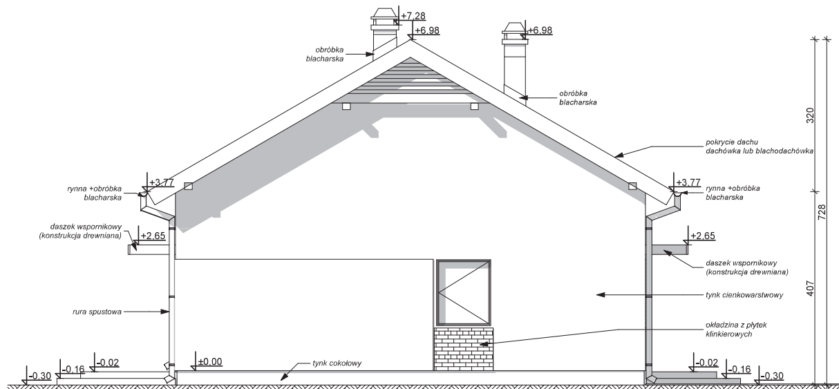
ELEWACJA BOCZNA
