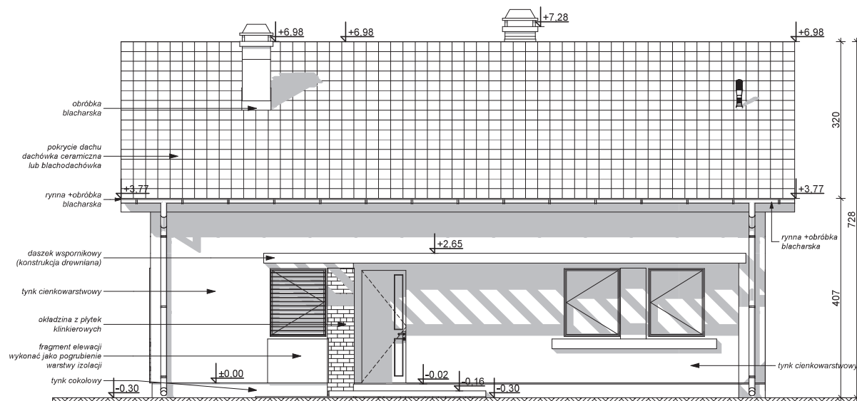
ELEWACJA FRONTOWA
