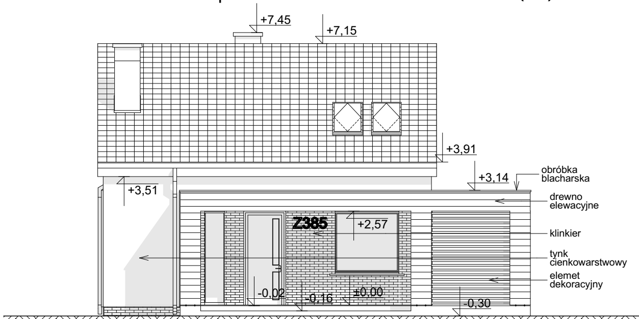
ELEWACJA FRONTOWA
