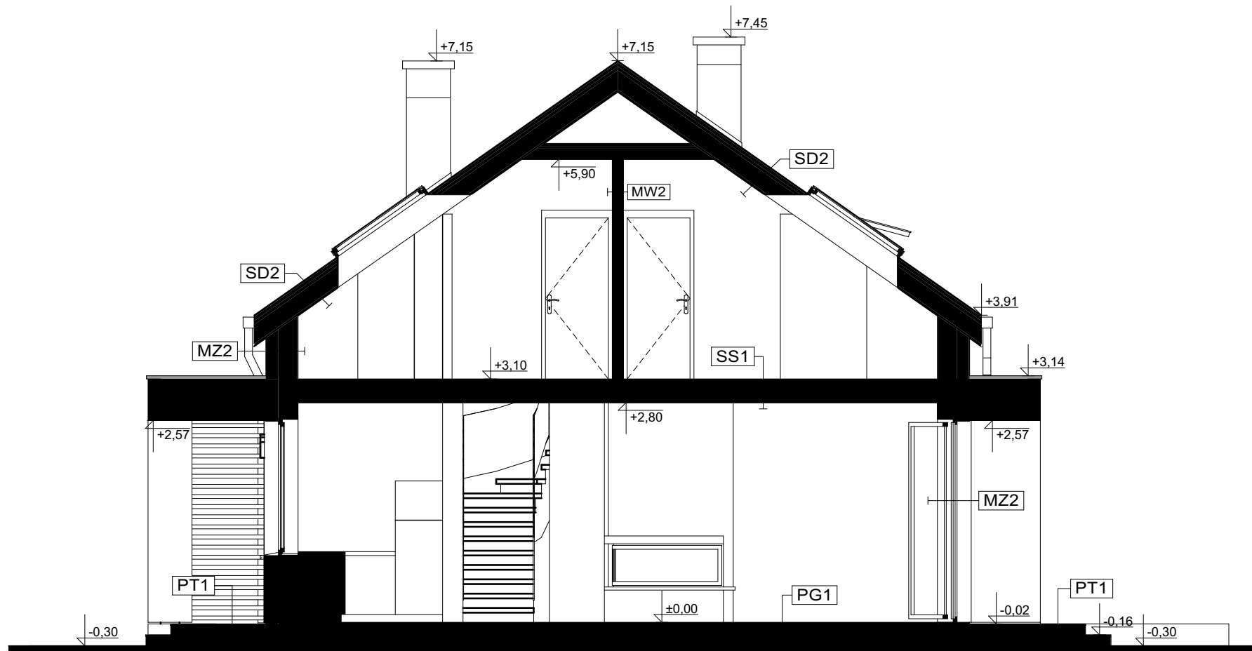
B-B PRZEKRÓJ
