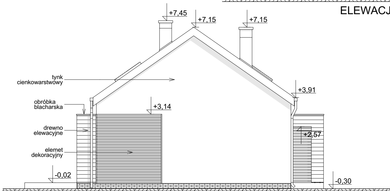
ELEWACJA BOCZNA
