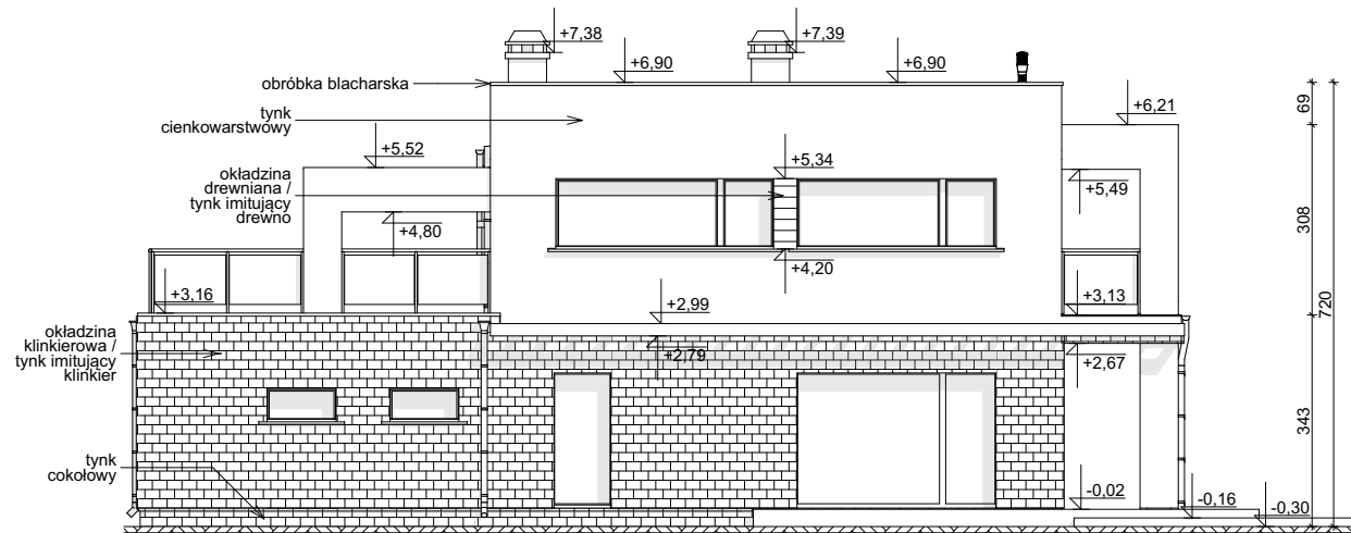
ELEWACJA OGRODOWA
