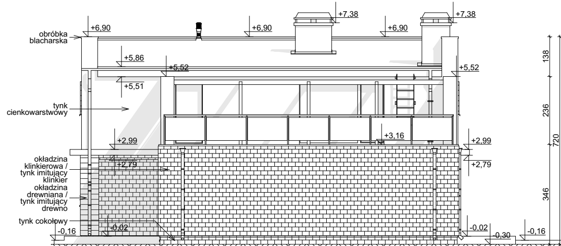
ELEWACJA BOCZNA
