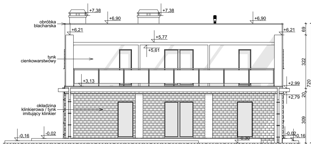
ELEWACJA BOCZNA
