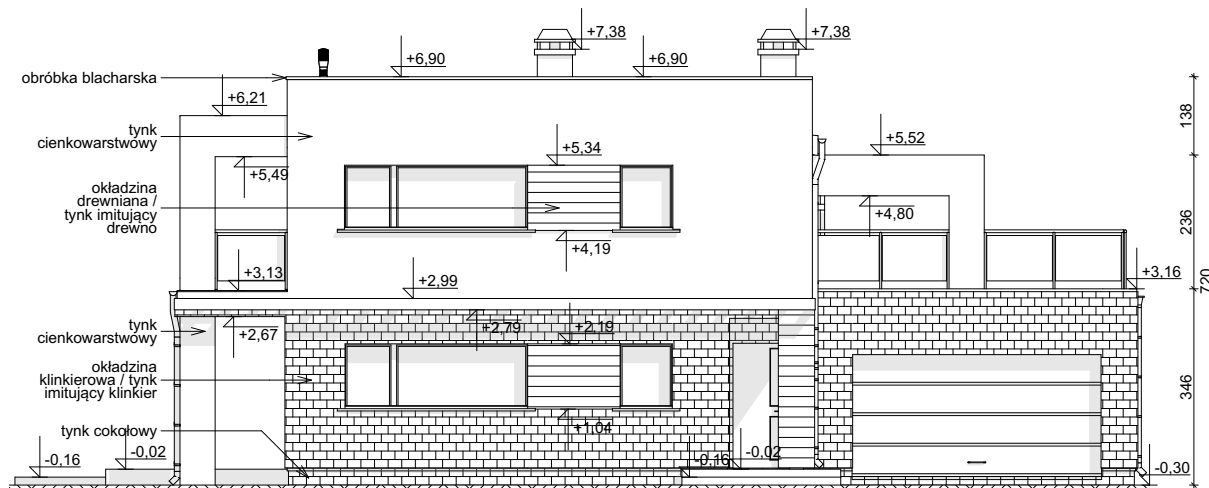
ELEWACJA FRONTOWA
