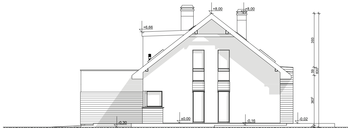
ELEWACJA BOCZNA
