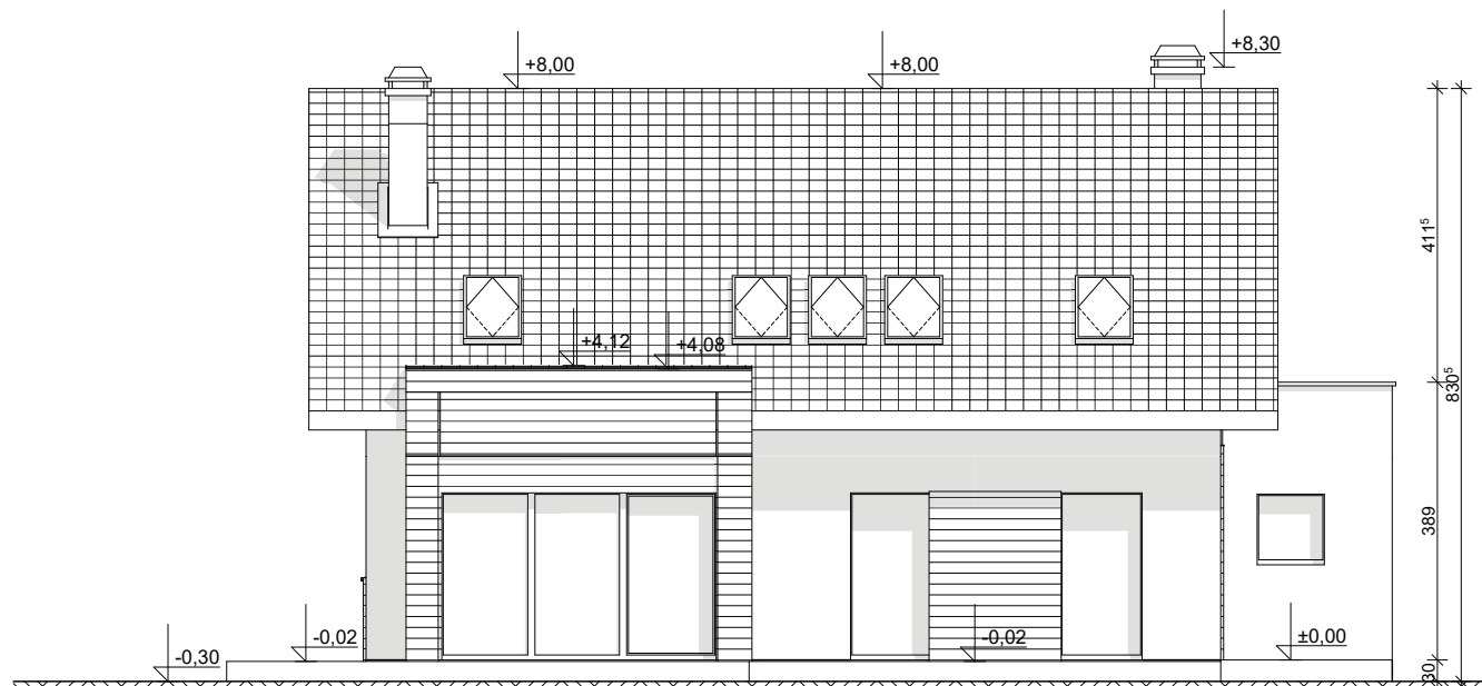
ELEWACJA OGRODOWA
