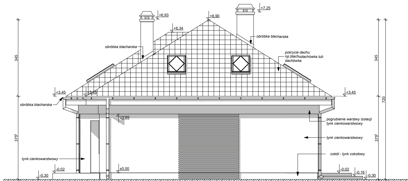
ELEWACJA BOCZNA
