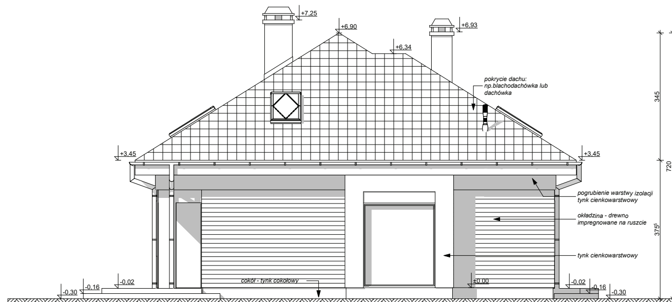
ELEWACJA BOCZNA
