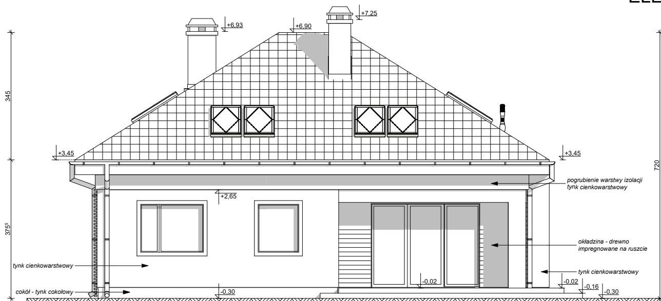
ELEWACJA OGRODOWA
