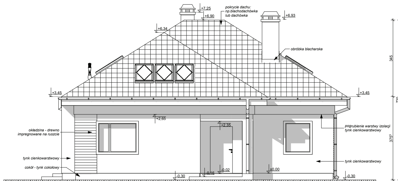
ELEWACJA FRONTOWA
