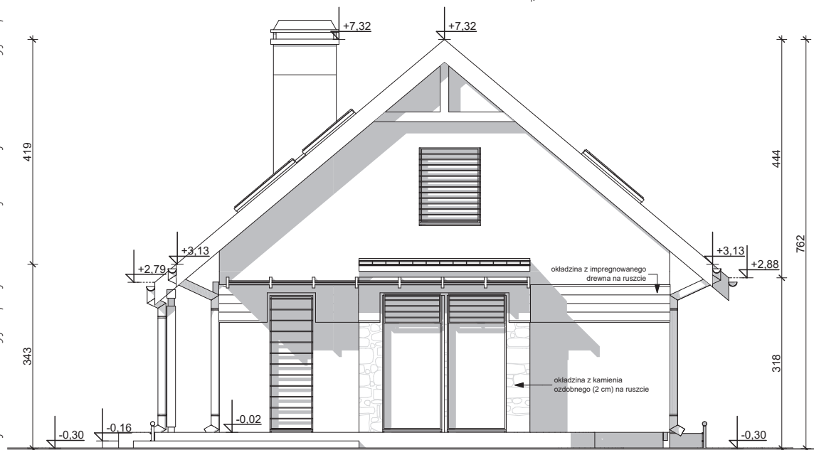
ELEWACJA BOCZNA
