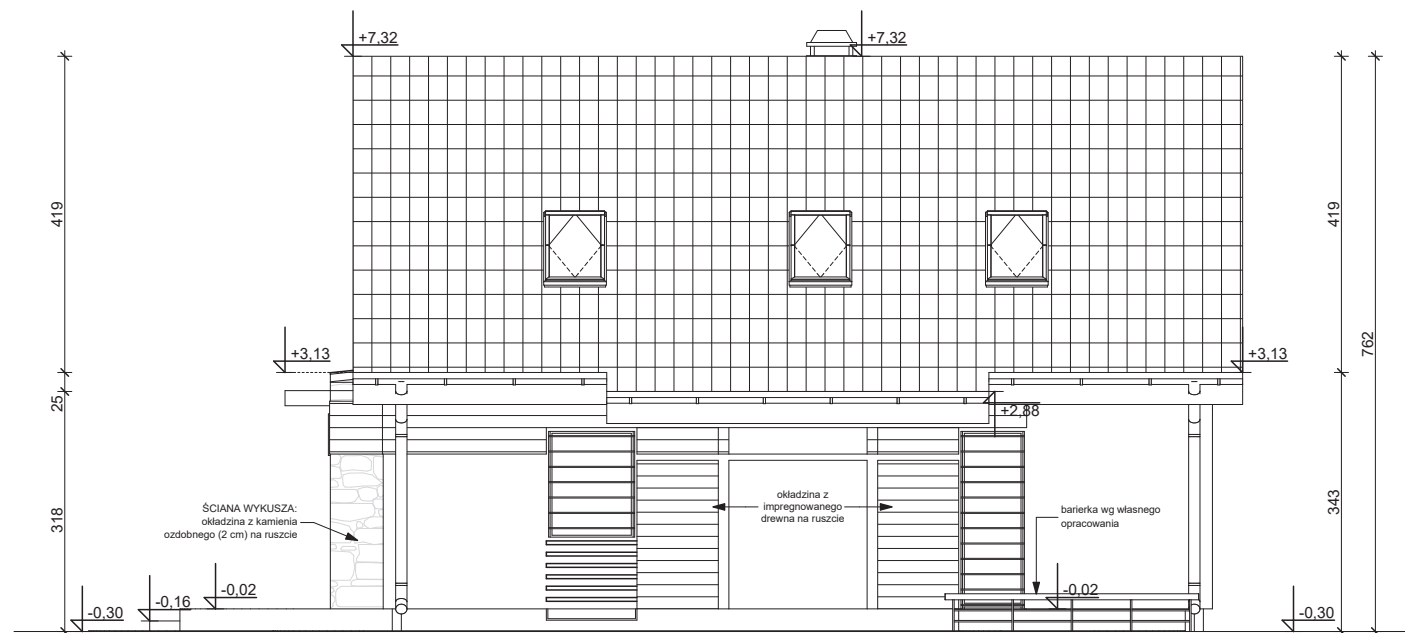
ELEWACJA TYLNA (ogrodowa)
