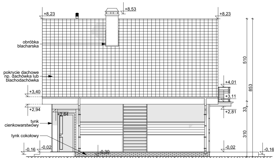
ELEWACJA BOCZNA
