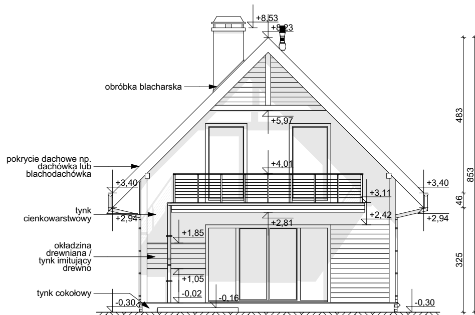
ELEWACJA OGRODOWA
