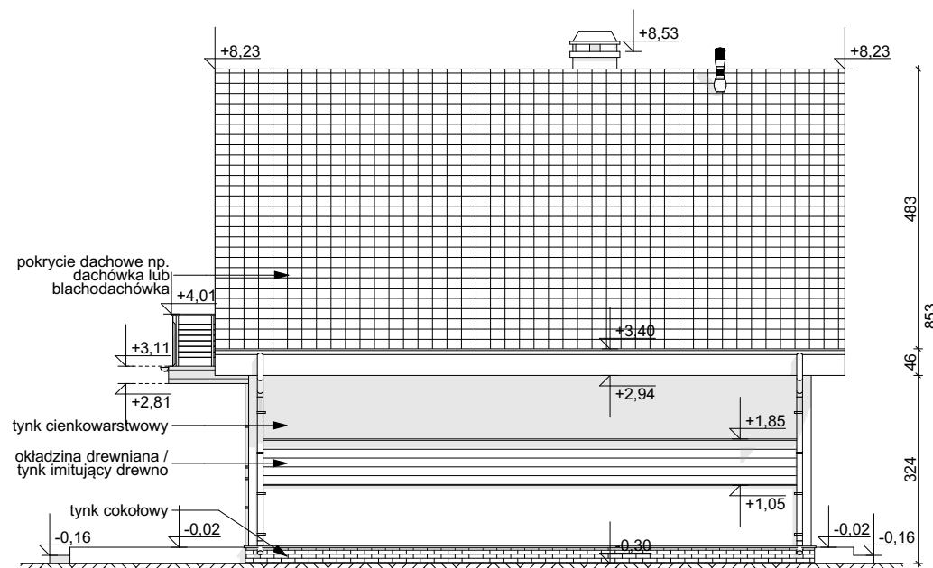
ELEWACJA BOCZNA
