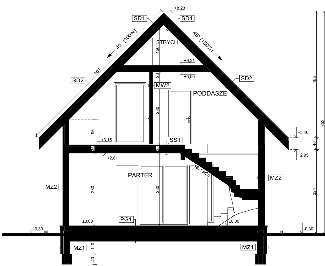
A-A PRZEKRÓJ
