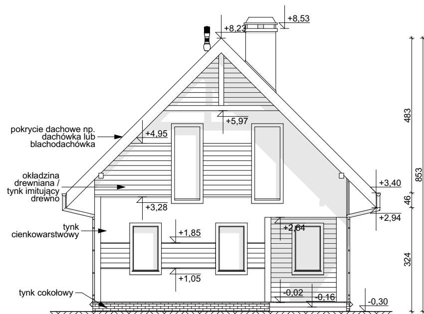
ELEWACJA FRONTOWA
