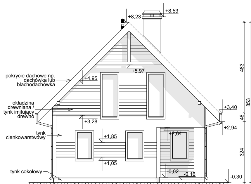
ELEWACJA FRONTOWA
