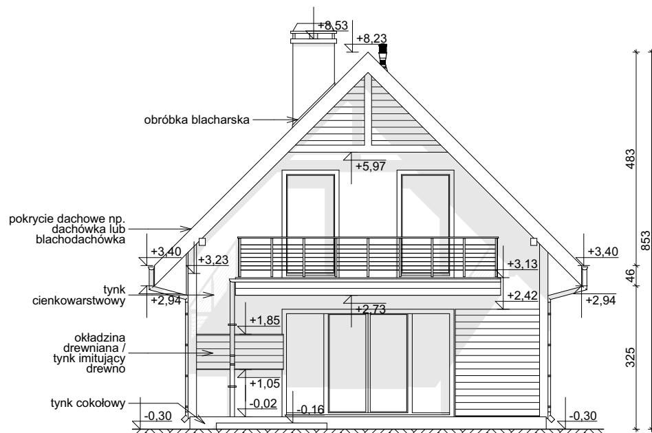
ELEWACJA OGRODOWA
