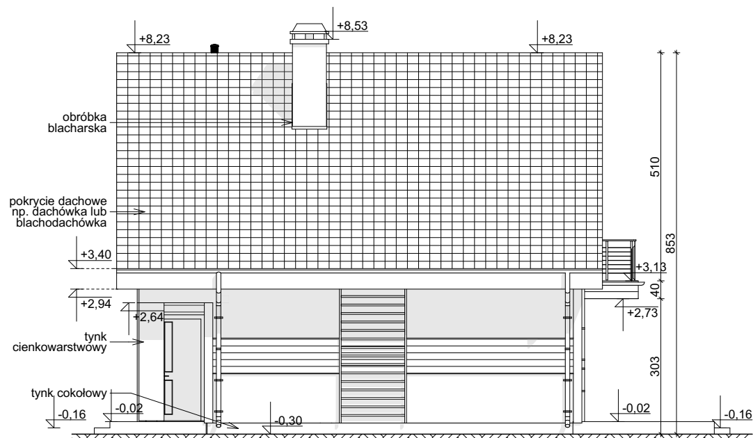
ELEWACJA BOCZNA
