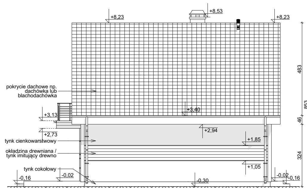
ELEWACJA BOCZNA
