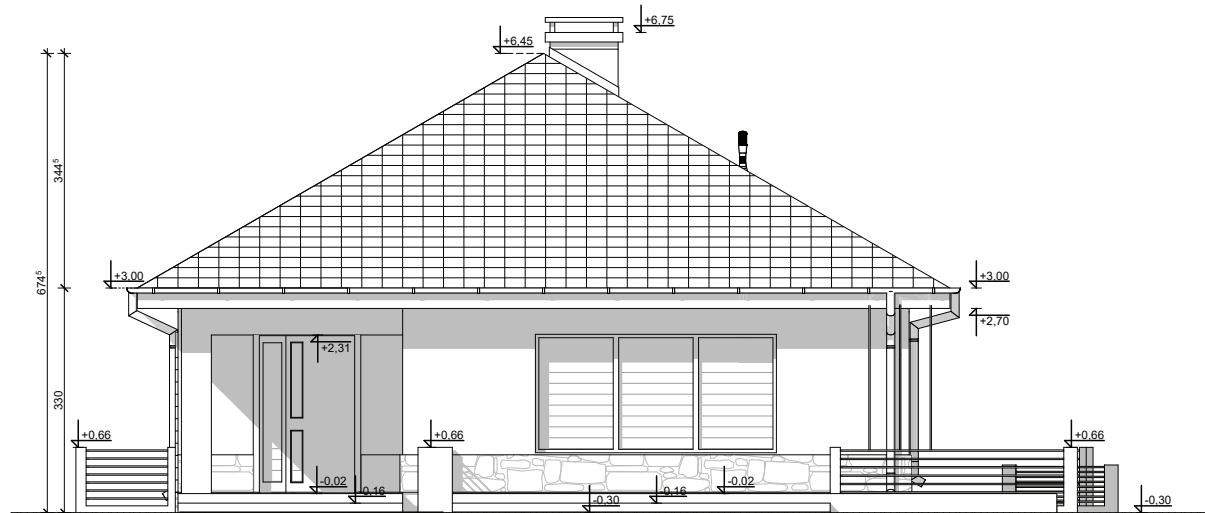
ELEWACJA FRONTOWA
