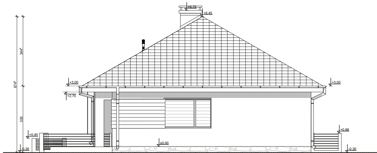
ELEWACJA TYLNA
