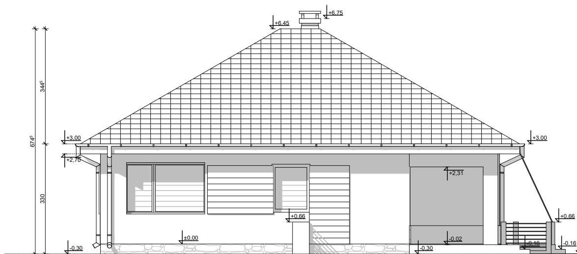
ELEWACJA BOCZNA
