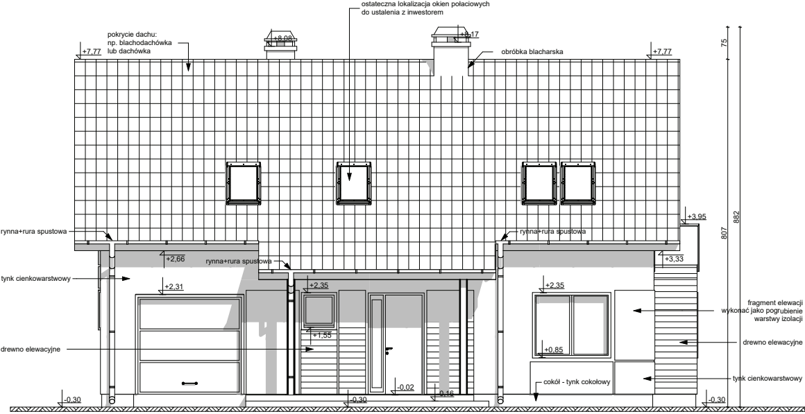
ELEWACJA FRONTOWA
