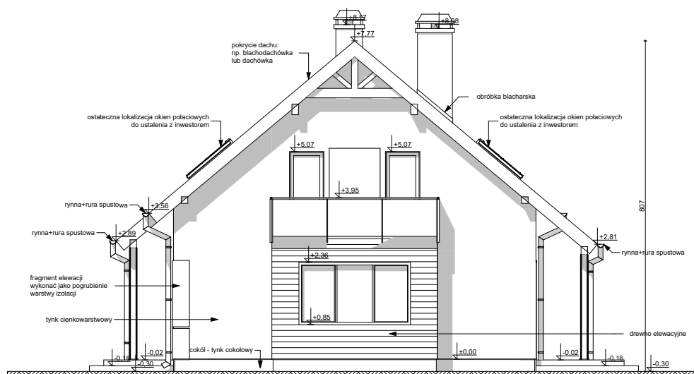
ELEWACJA BOCZNA
