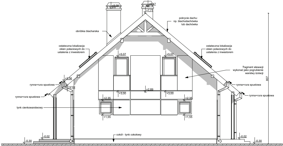
ELEWACJA BOCZNA
