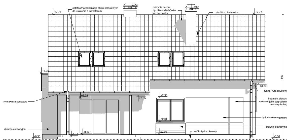
ELEWACJA OGRODOWA
