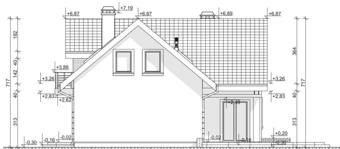
ELEWACJA BOCZNA
