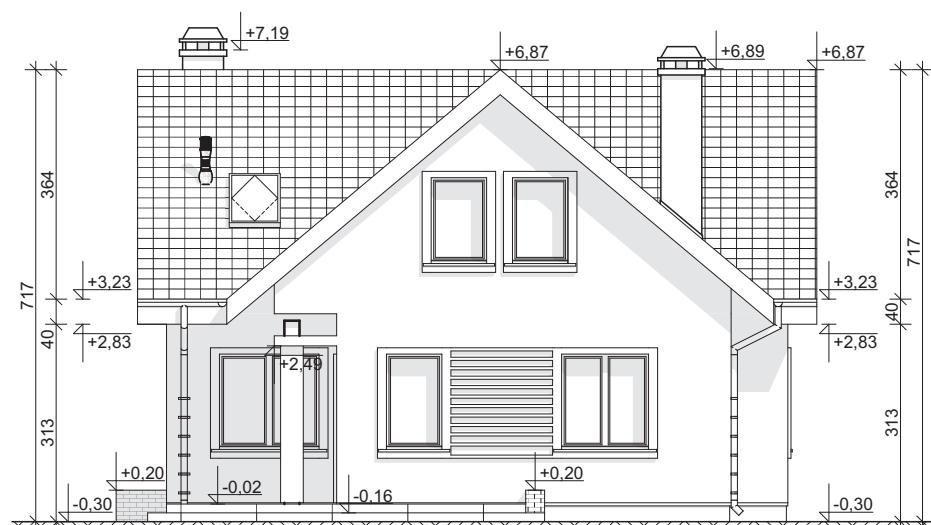
ELEWACJA OGRODOWA
