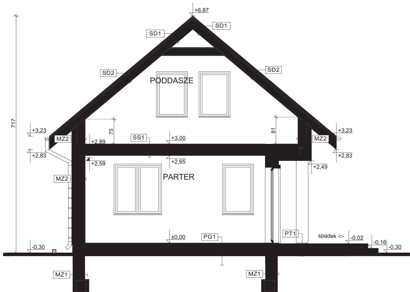
PRZEKRÓJ A-A
