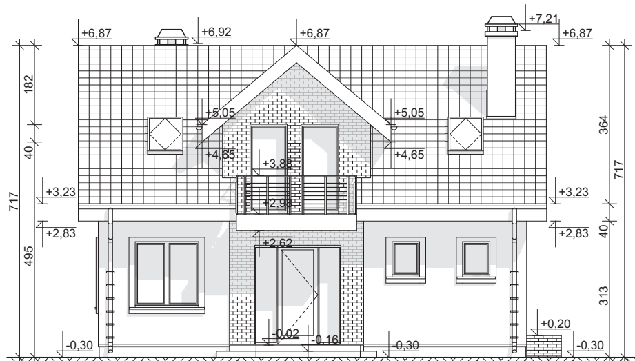
ELEWACJA FRONTOWA
