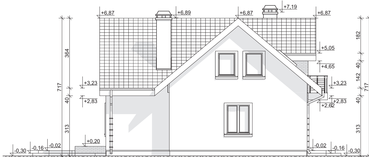
ELEWACJA BOCZNA
