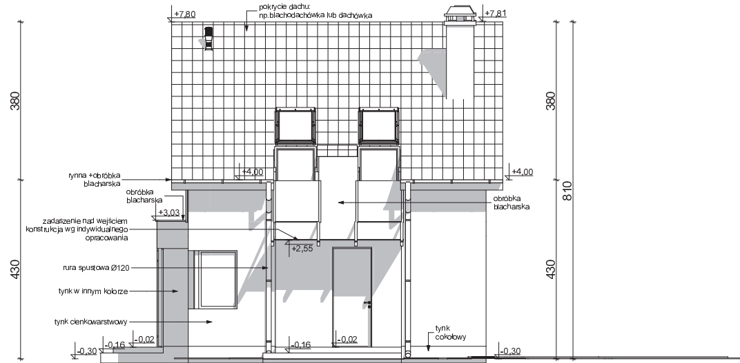
ELEWACJA FRONTOWA
