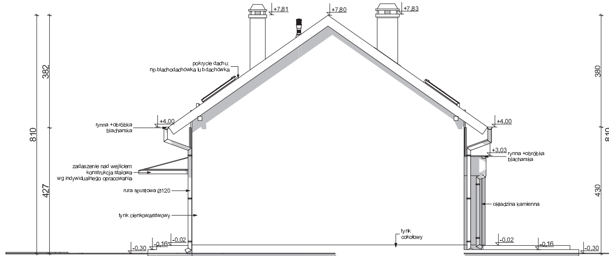
ELEWACJA BOCZNA
