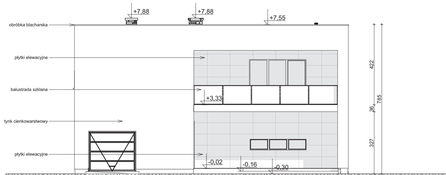
ELEWACJA FRONTOWA
