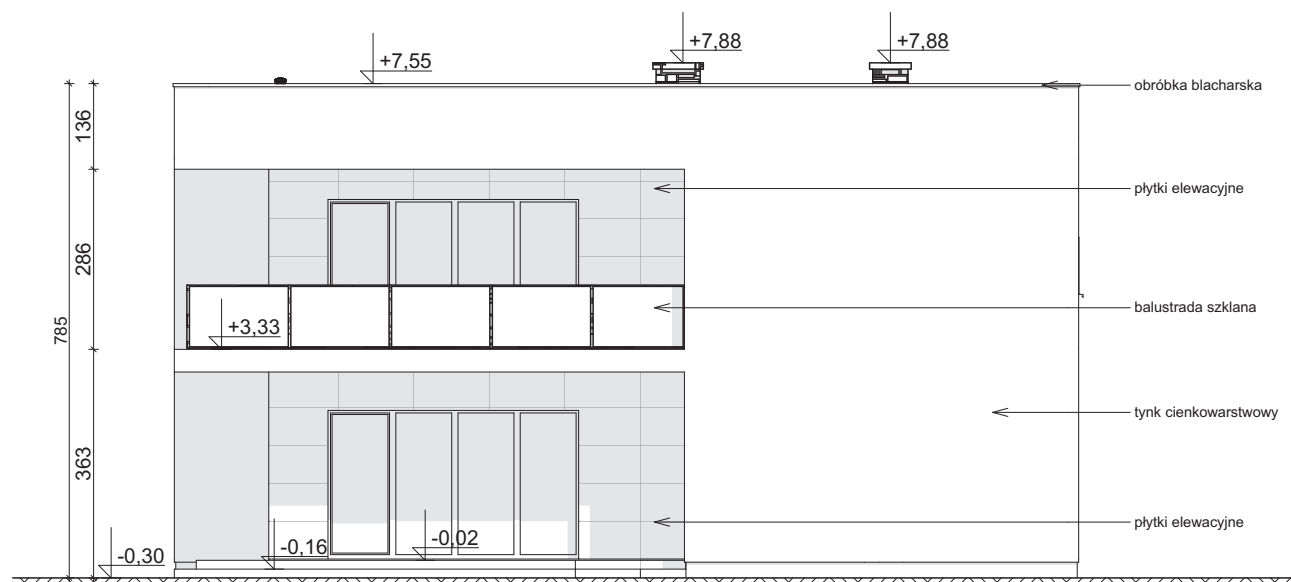
ELEWACJA OGRODOWA
