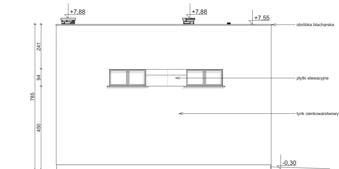
ELEWACJA BOCZNA
