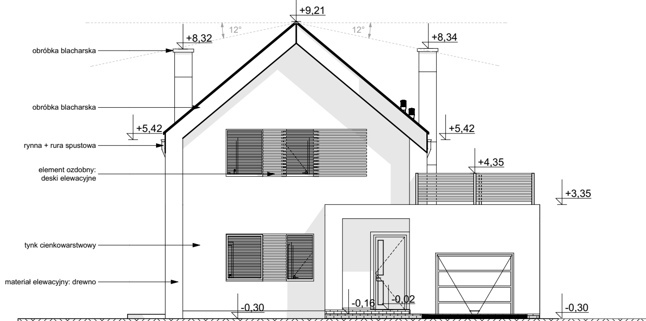
ELEWACJA FRONTOWA
