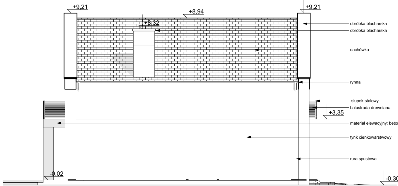
ELEWACJA BOCZNA
