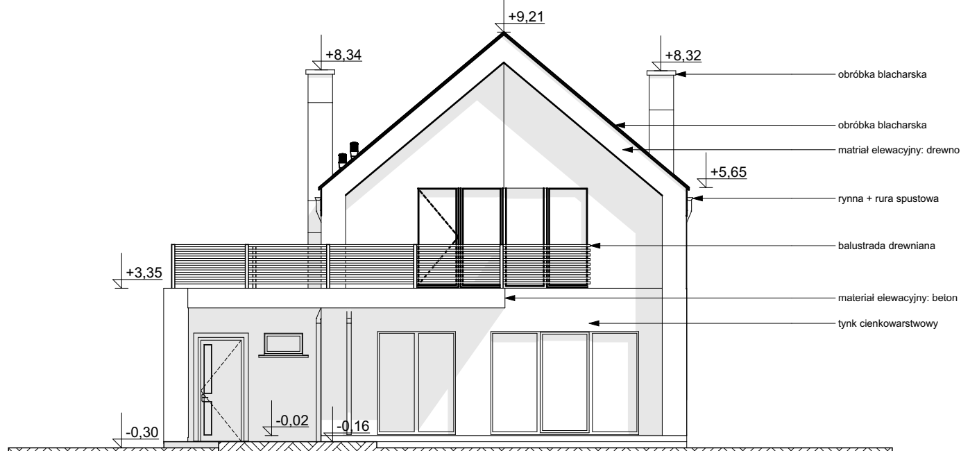
ELEWACJA OGRODOWA
