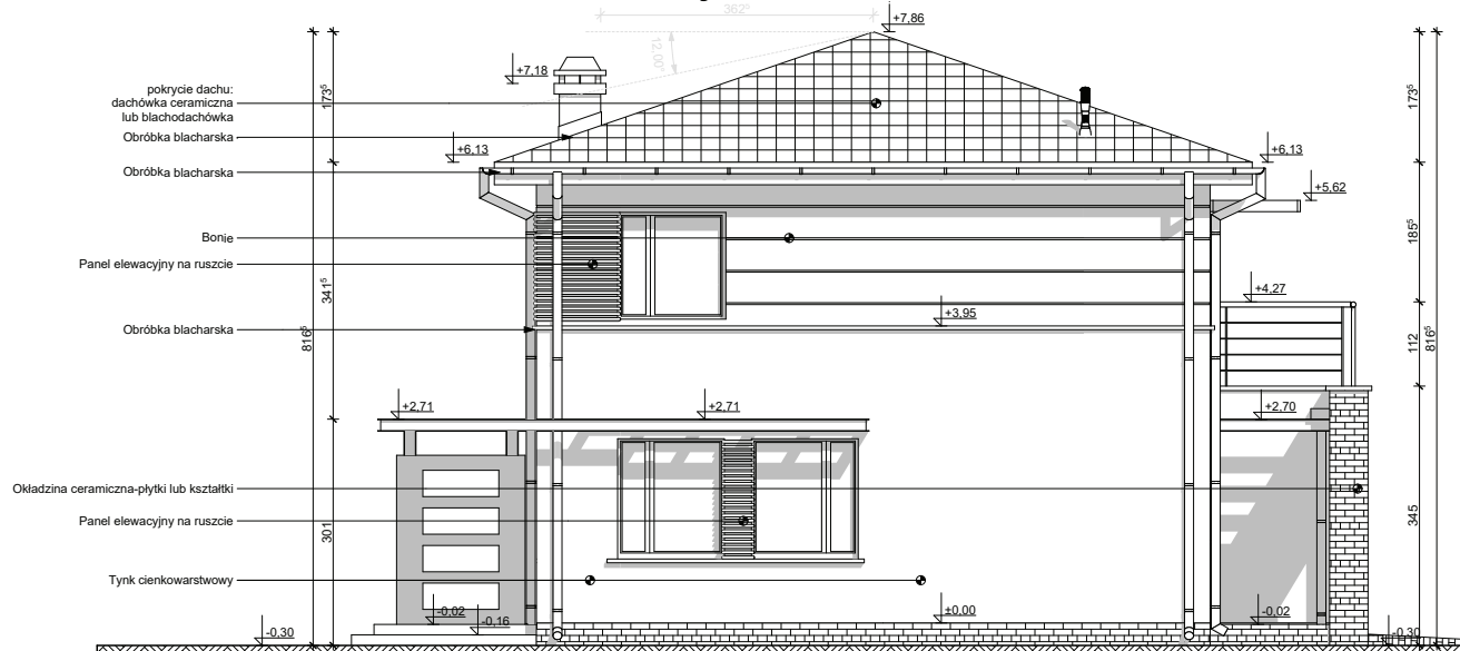
Elewacja boczna
