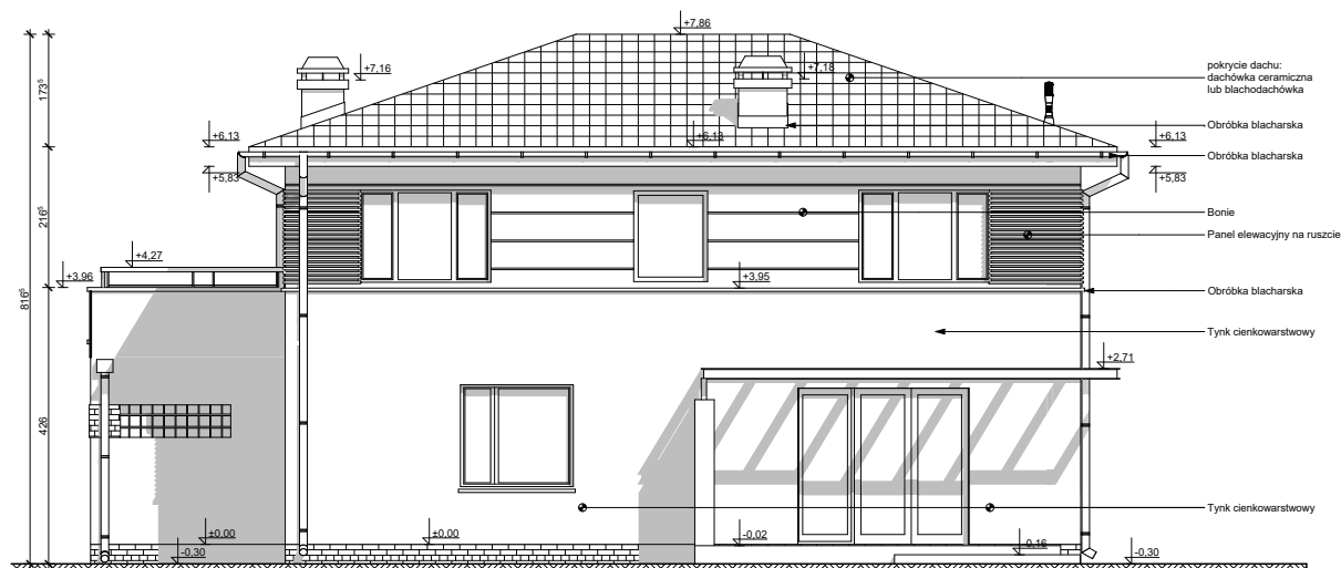
Elewacja tylna
