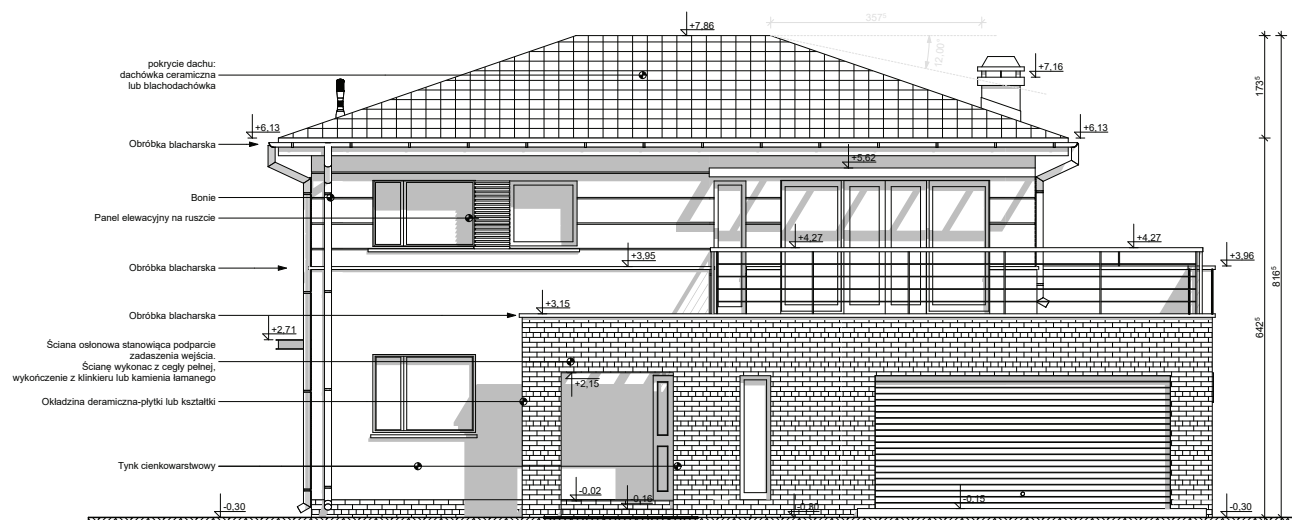
Elewacja front
