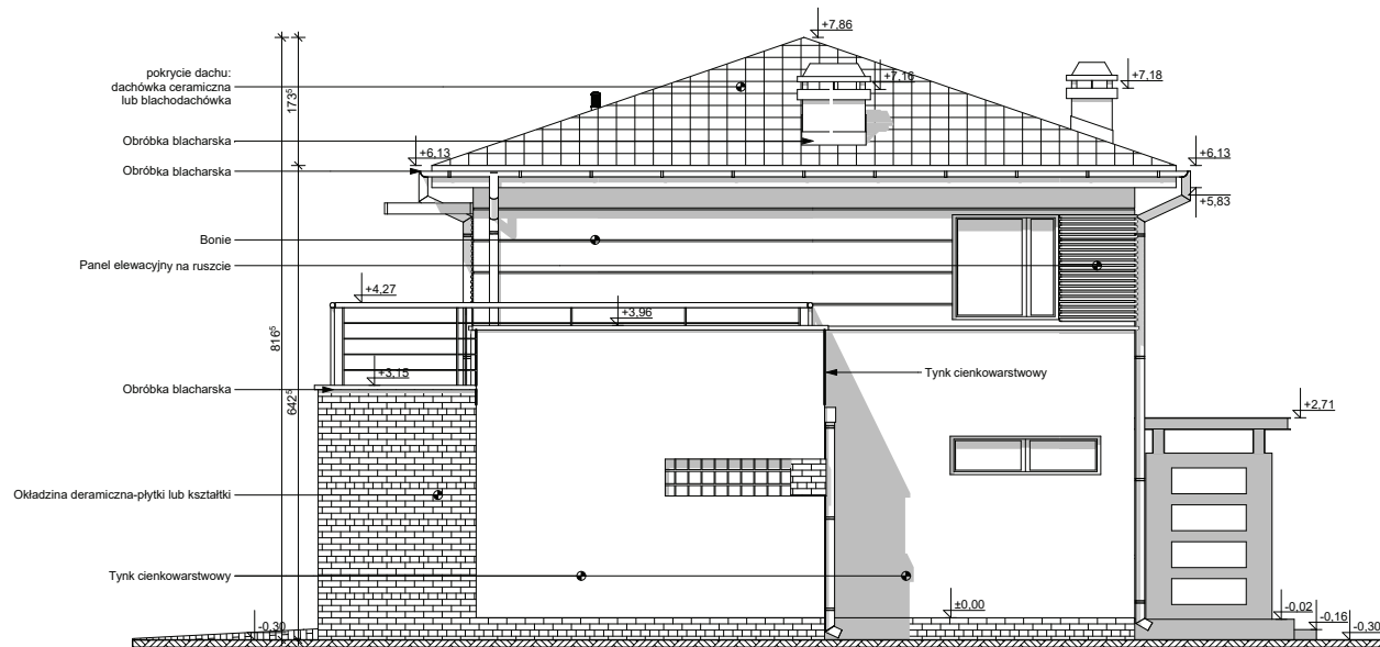
Elewacja boczna
