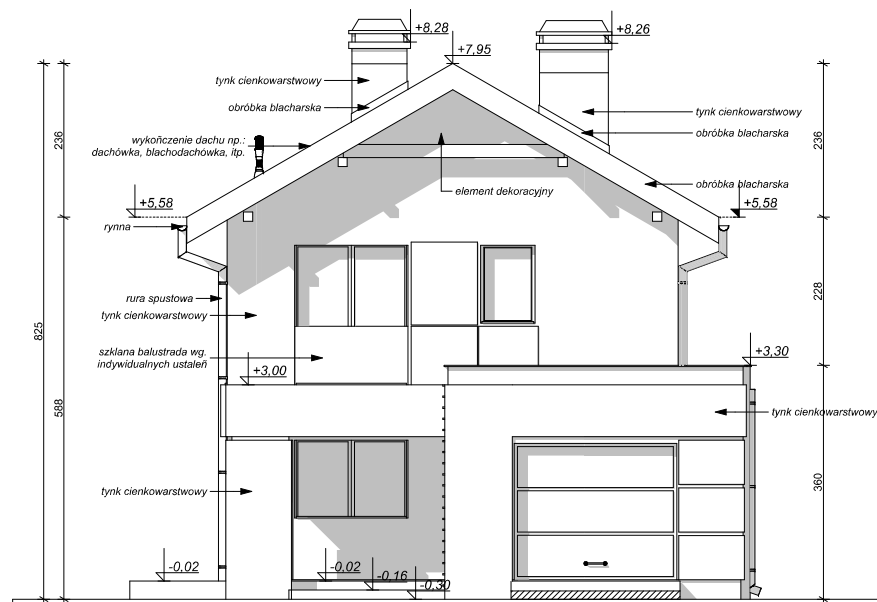
ELEWACJA FRONTOWA
