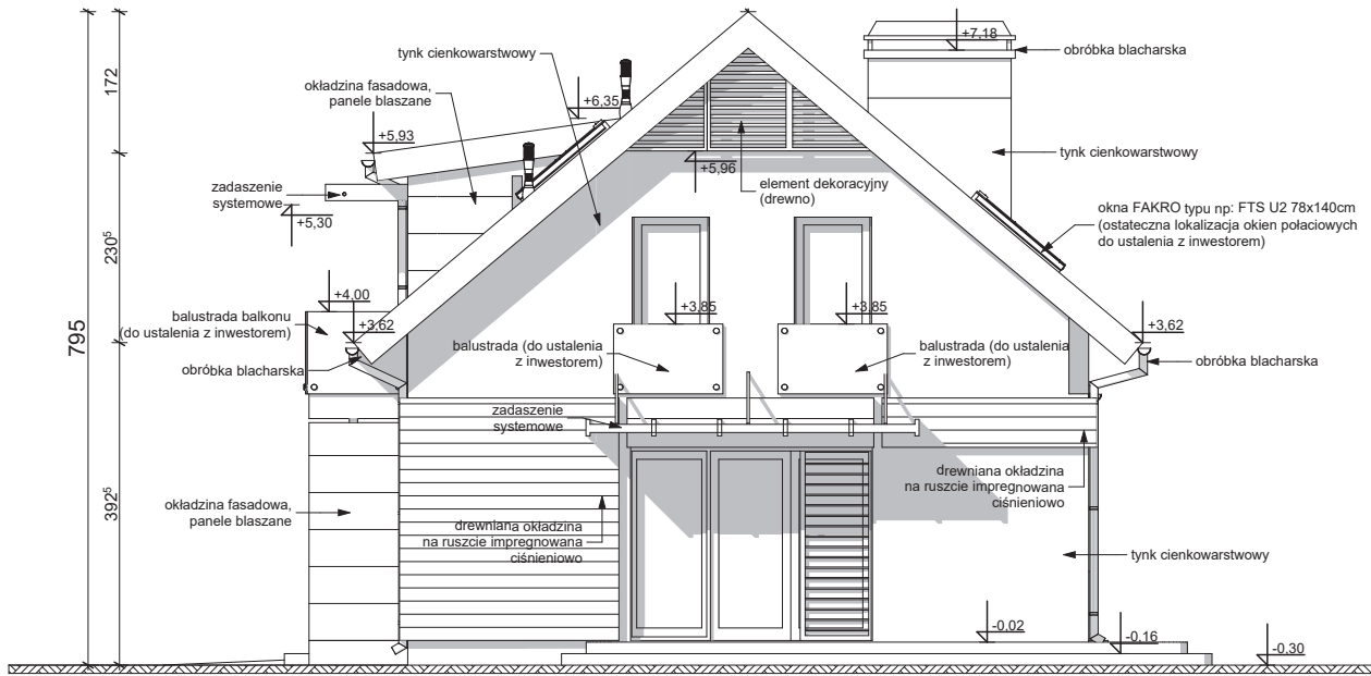
ELEWACJA BOCZNA
