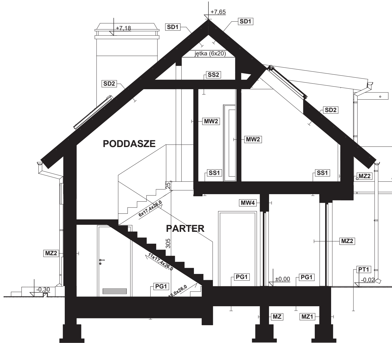
PRZEKRÓJ B-B
