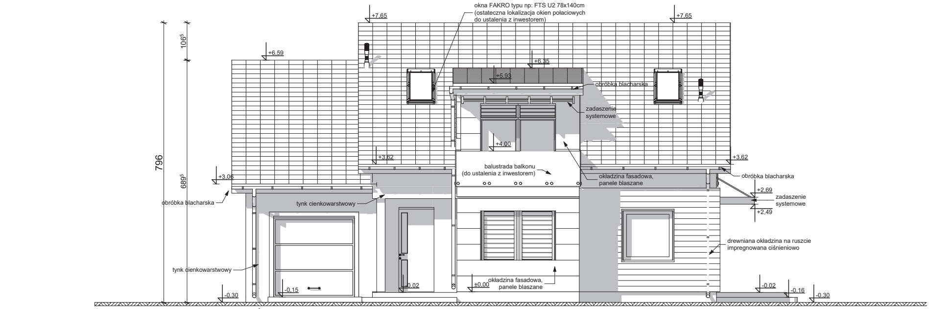
ELEWACJA FRONTOWA
