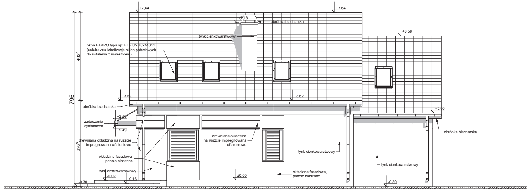
ELEWACJA TYLNA
