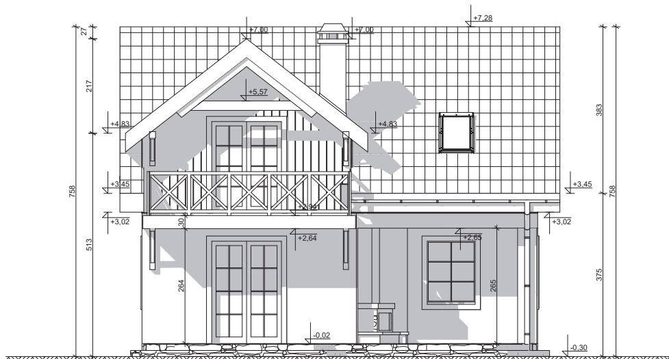
ELEWACJA TYLNA
