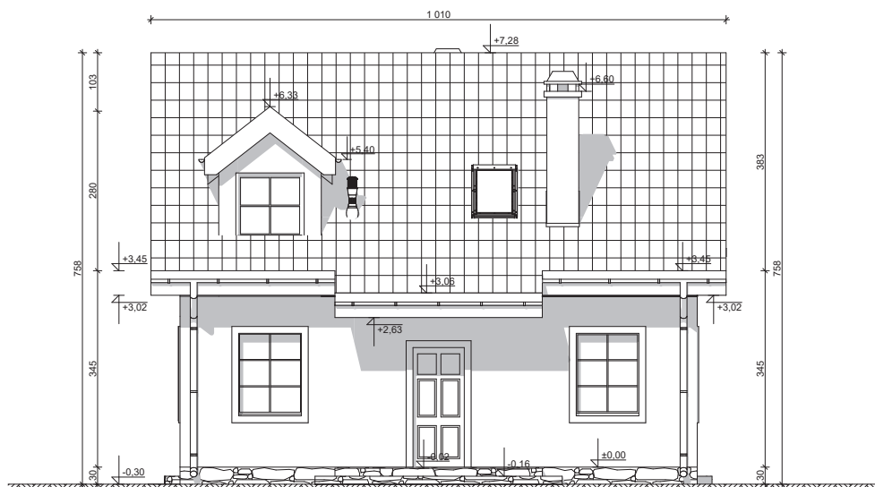
ELEWACJA FRONTOWA
