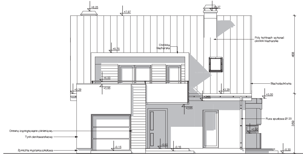
ELEWACJA FRONTOWA
