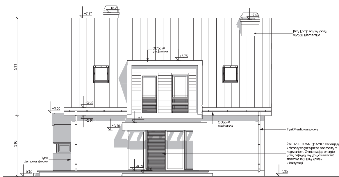
ELEWACJA OGRODOWA
