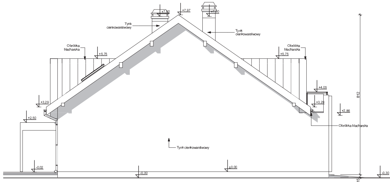
ELEWCJA BOCZNA
