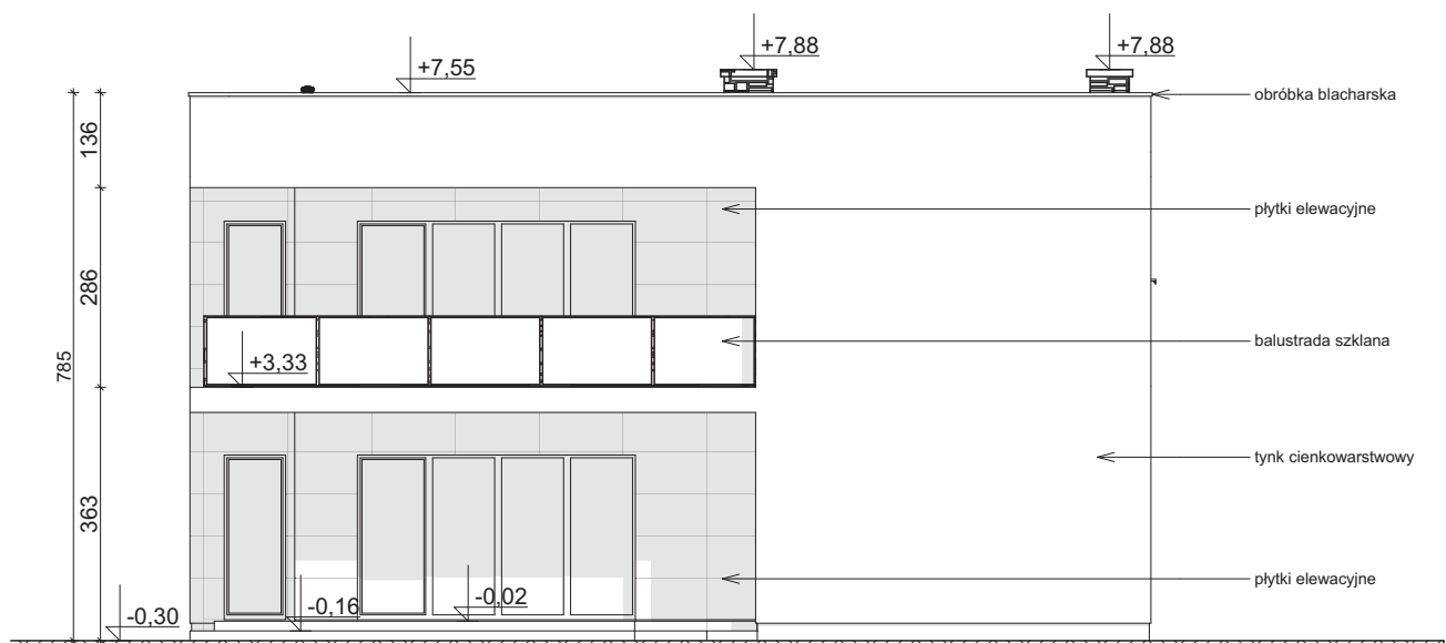
ELEWACJA OGRODOWA
