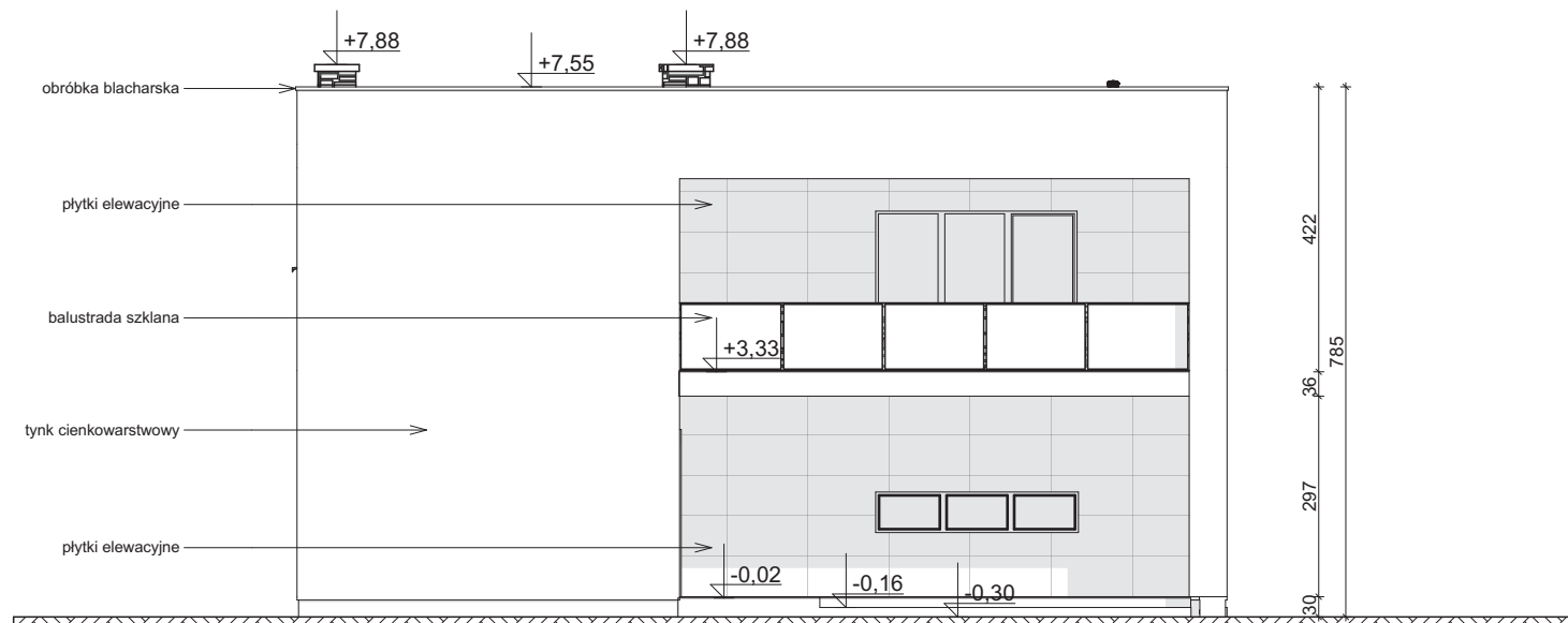
ELEWACJA FRONTOWA
