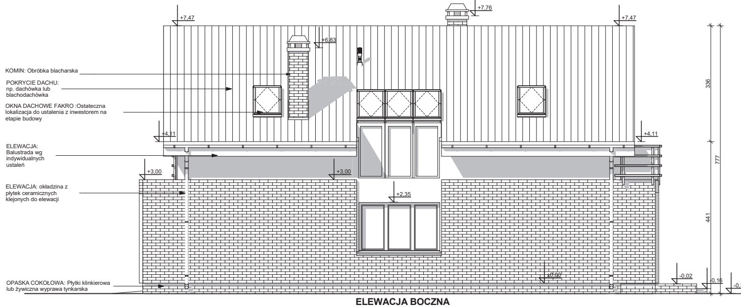
ELEWACJA BOCZNA
