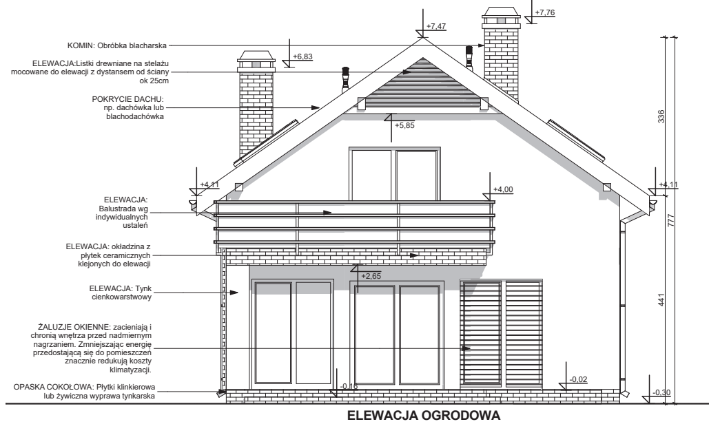
ELEWACJA OGRODOWA
