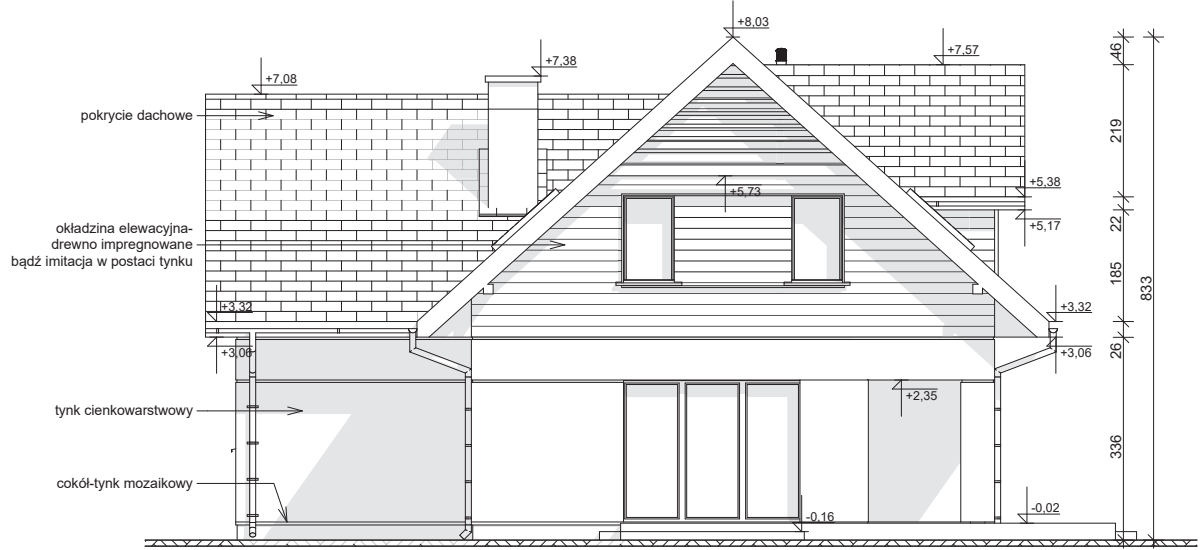
ELEWACJA BOCZNA
