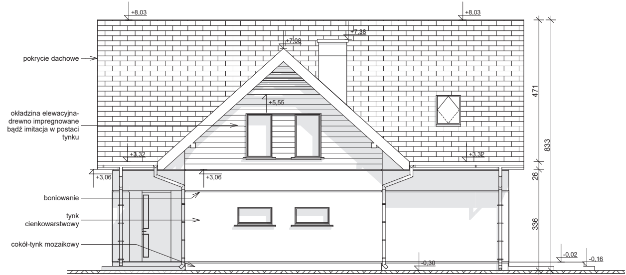
ELEWACJA FRONTOWA
