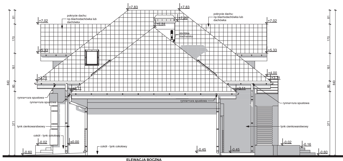
ELEWACJA BOCZNA
