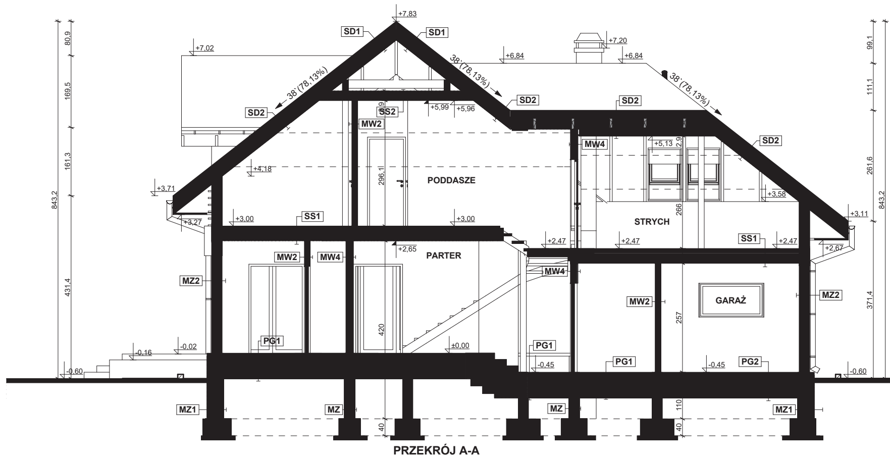
PRZEKRÓJ A-A
