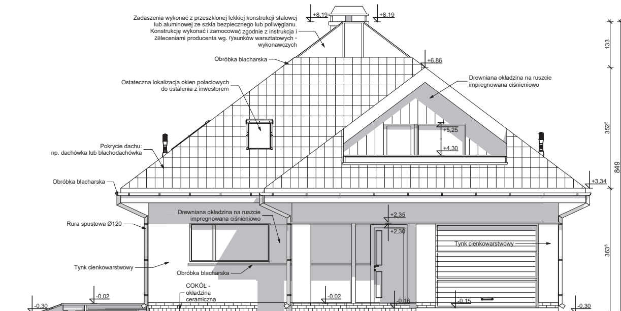
ELEWACJA FRONTOWA
