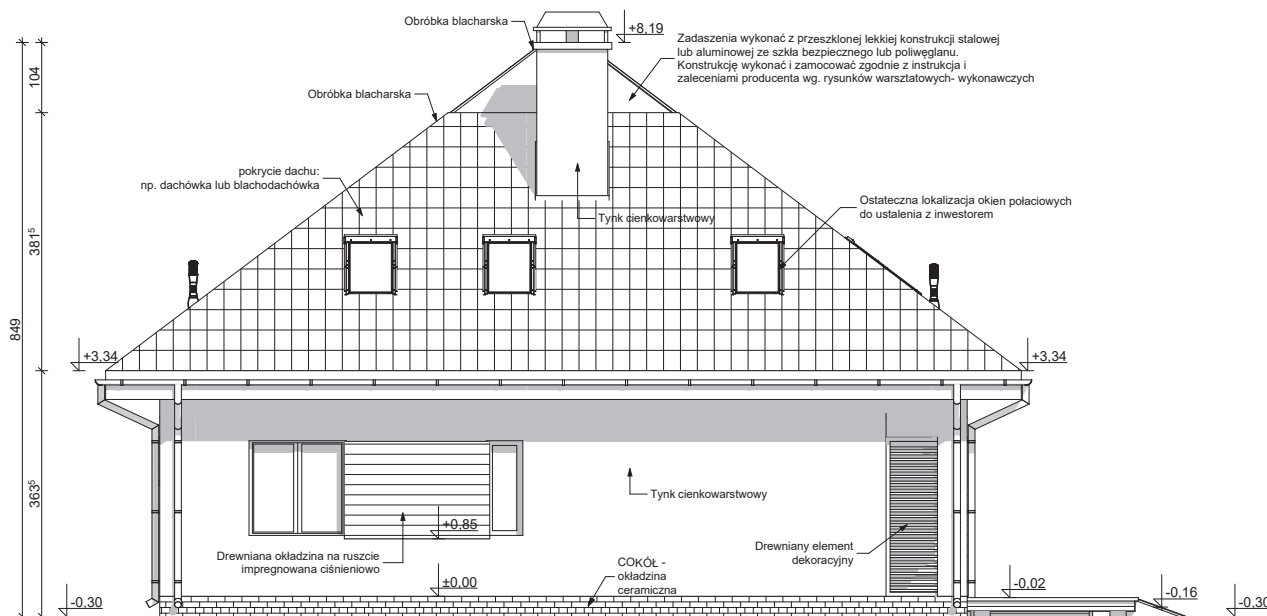
ELEWACJA OGRODOWA
