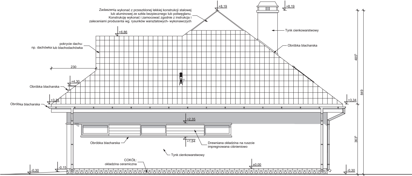
ELEWACJA BOCZNA
