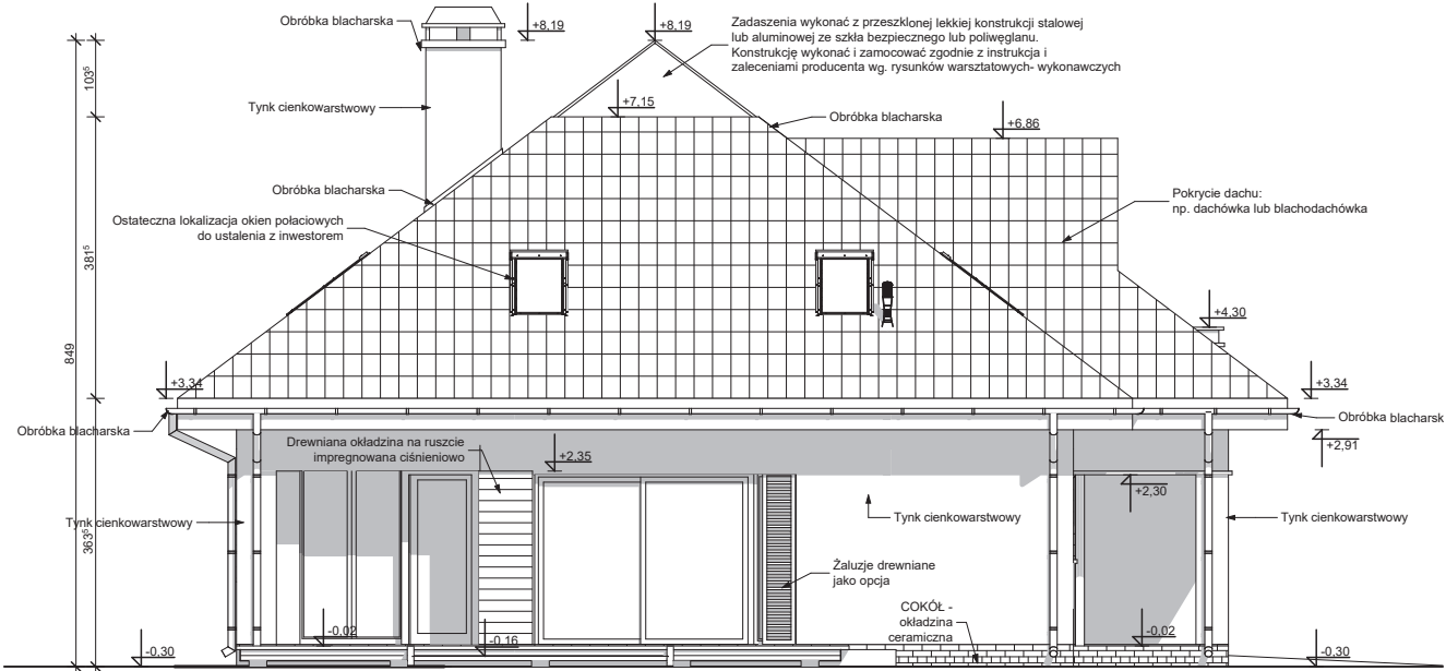
ELEWACJA BOCZNA
