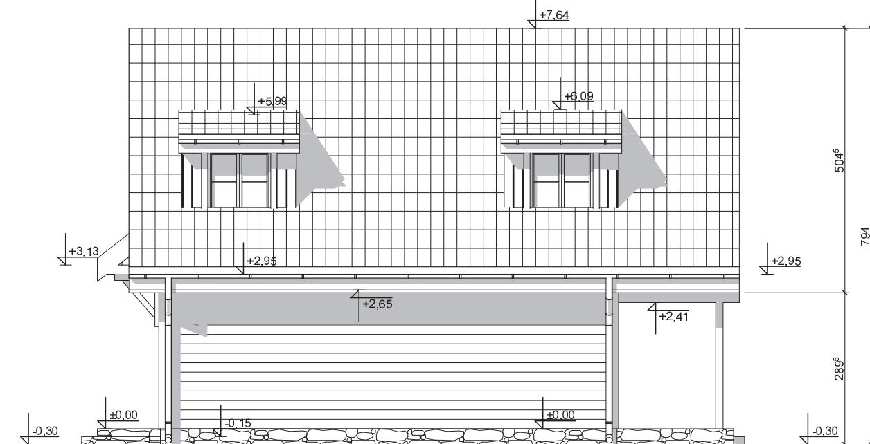
ELEWACJA BOCZNA
