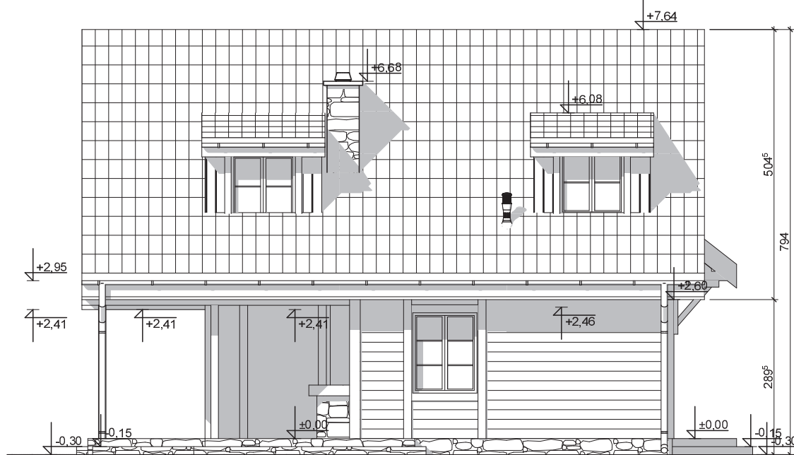
ELEWACJA BOCZNA
