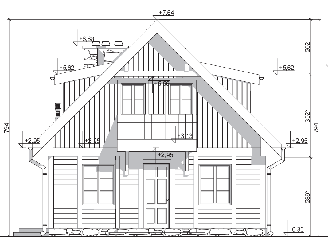
ELEWACJA FRONTOWA
