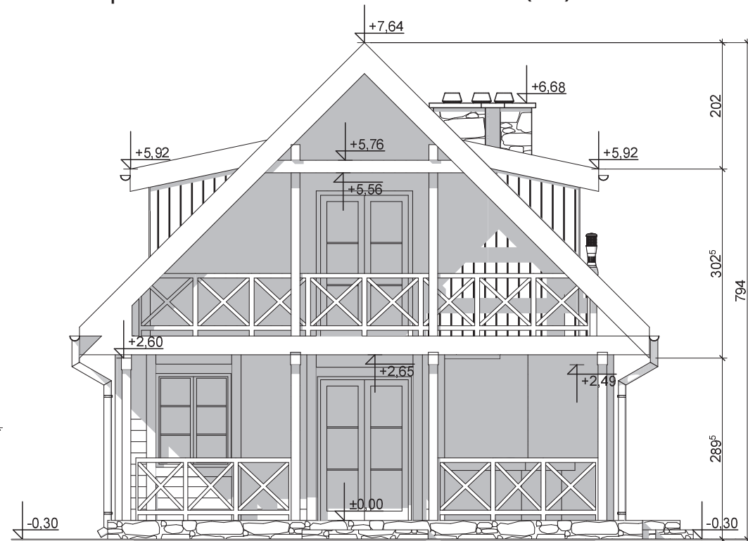
ELEWACJA OGRODOWA
