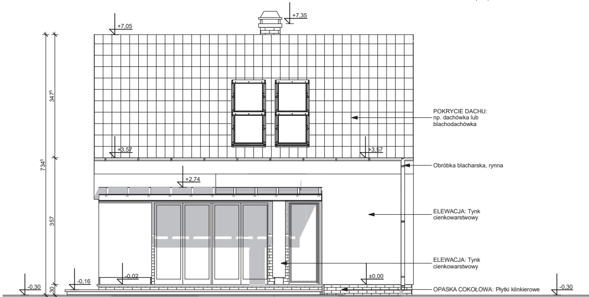
ELEWACJA TYLNA
