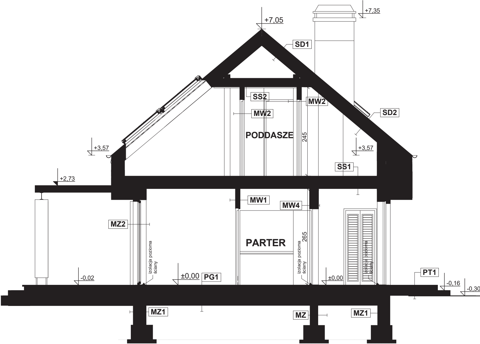
PRZEKRÓJ A-A
