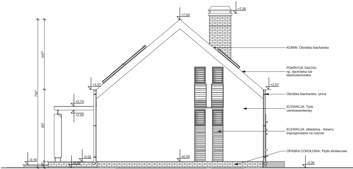
ELEWACJA BOCZNA
