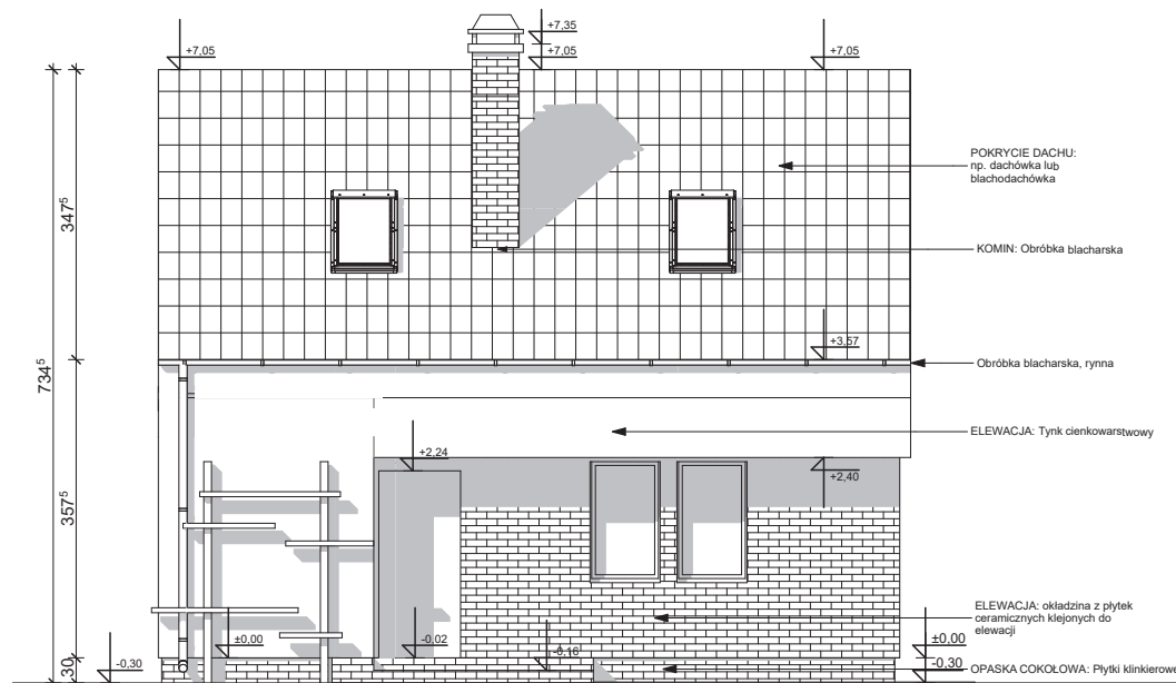
ELEWACJA FRONTOWA
